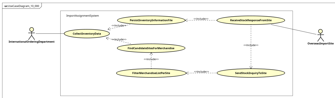
Figure 3.1: Use case phân rã UC003 - CollectInventoryData
