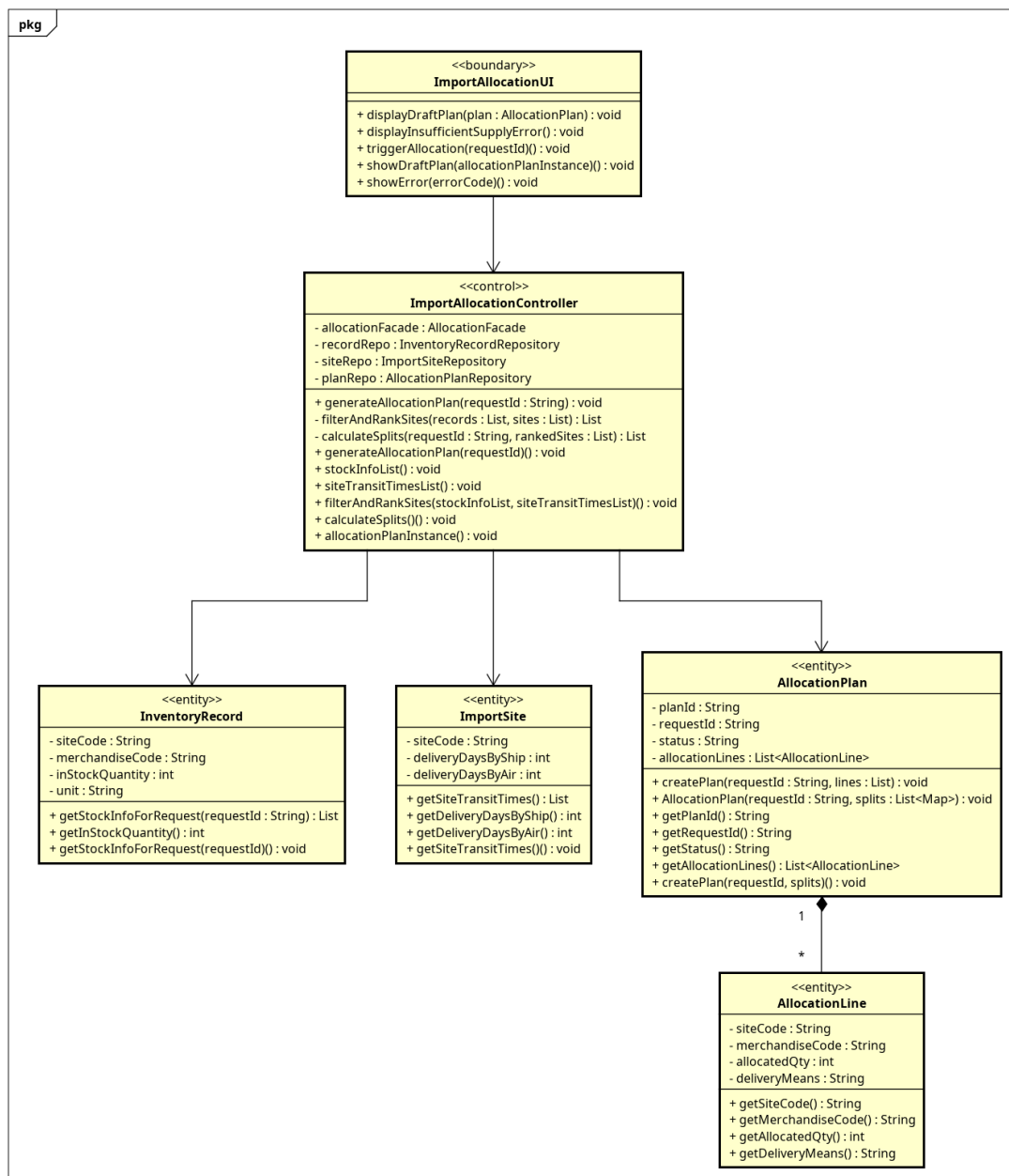
Figure 3.13: Class diagram mức phân tích UC004 - PlanImportAllocation
