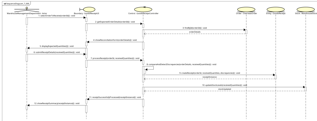
Figure 3.17: Sequence diagram mức phân tích UC006 - ReceiveAndReconcileGoods
