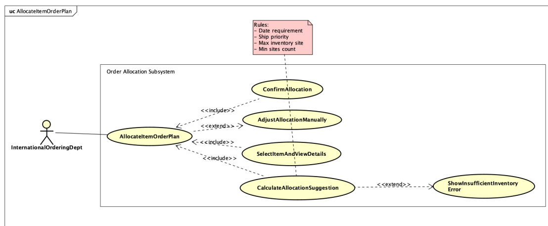
Hình 1: Biểu đồ Use case Phân rã cho UC005
