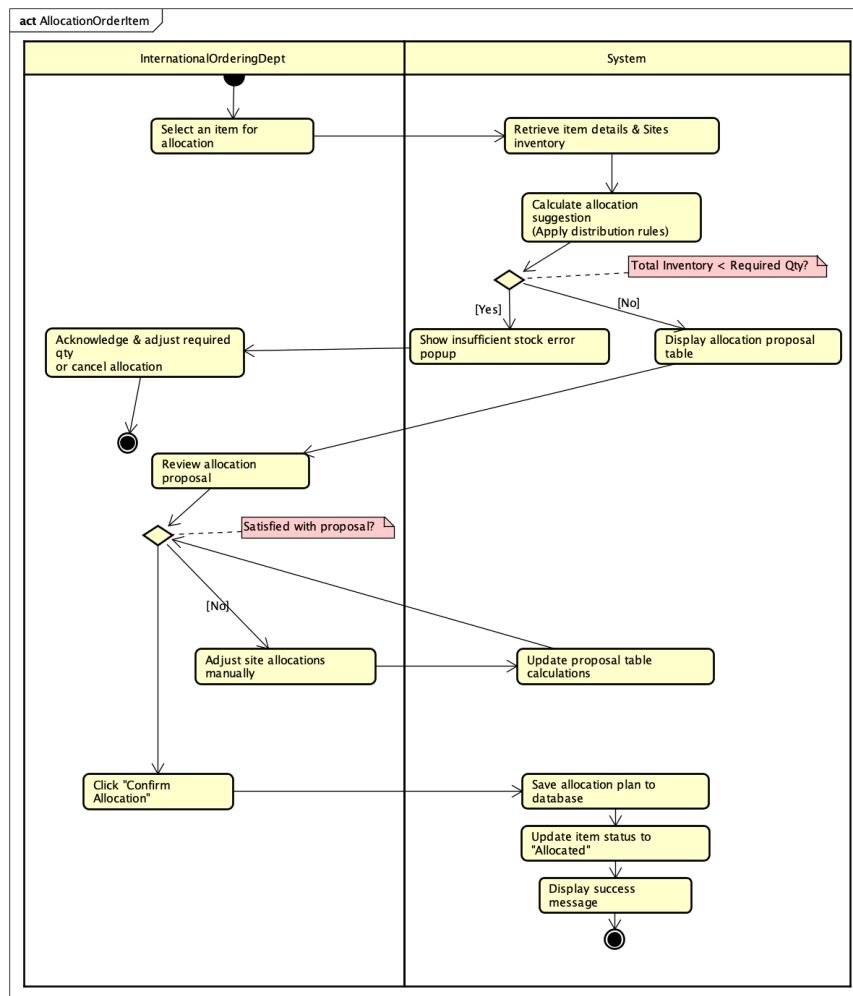
Hình 2: Biểu đồ Hoạt động cho UC005 - Phân bổ phương án đặt hàng
