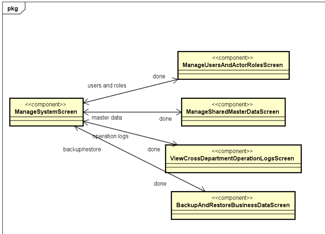
Hình 4.8: Sơ đồ màn hình ManageSystem.
