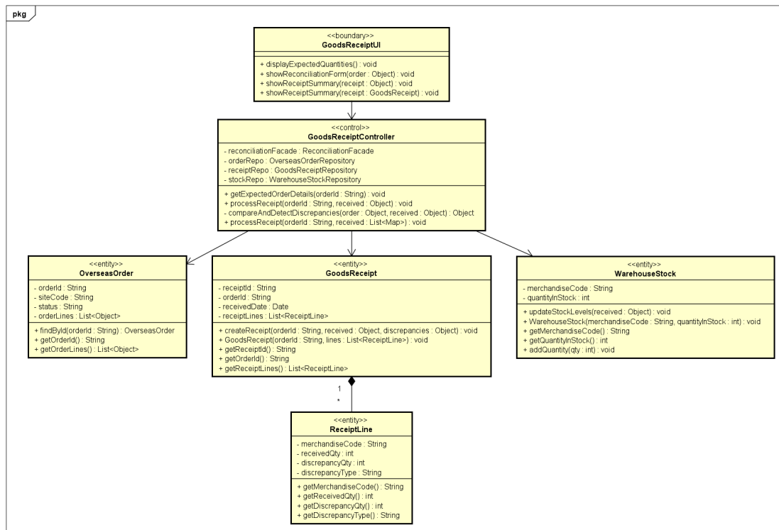
Hình 3.19: Lớp phân tích của ReceiveAndReconcileGoods .
