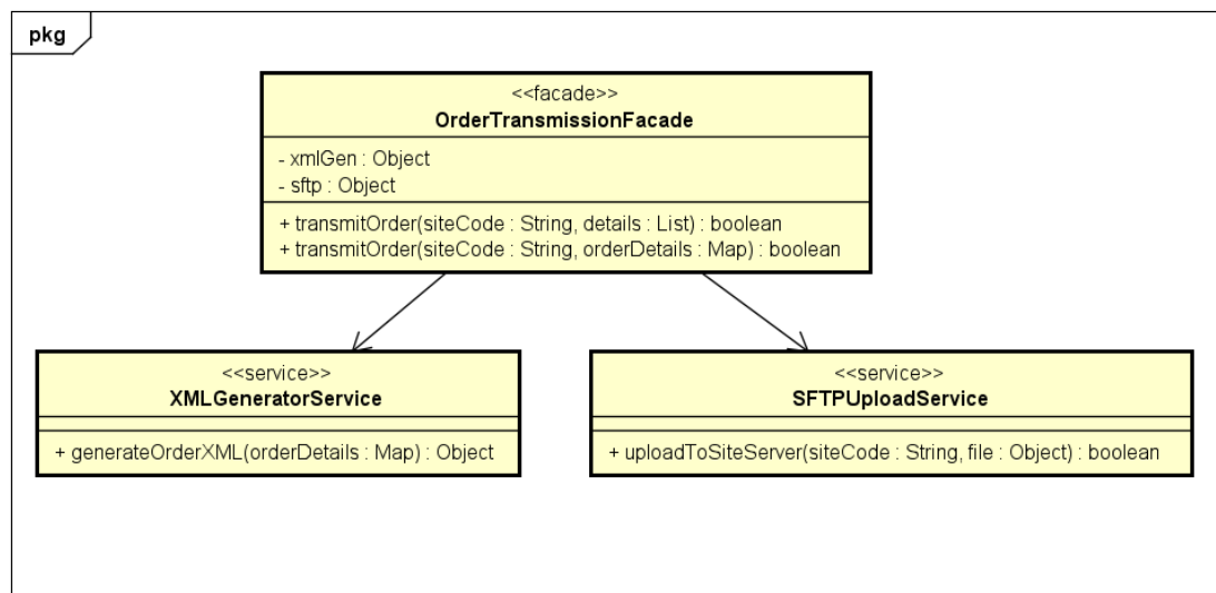
Hình 5.5: Subsystem truyền đơn đặt hàng cho PlaceOverseasOrders.
