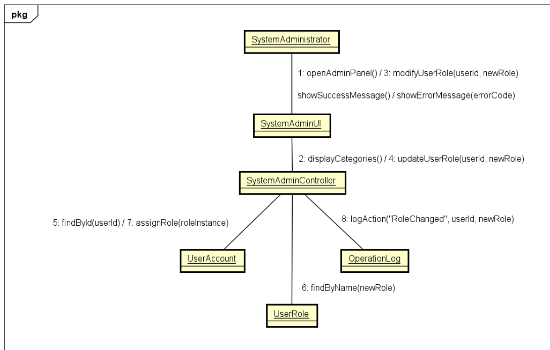
Hình 3.21: Communication phân tích của ManageSystem.
