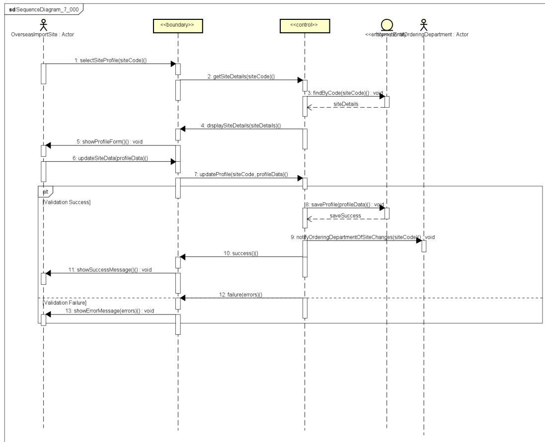
Hình 3.5: Sequence phân tích của ManageSiteInformation.
