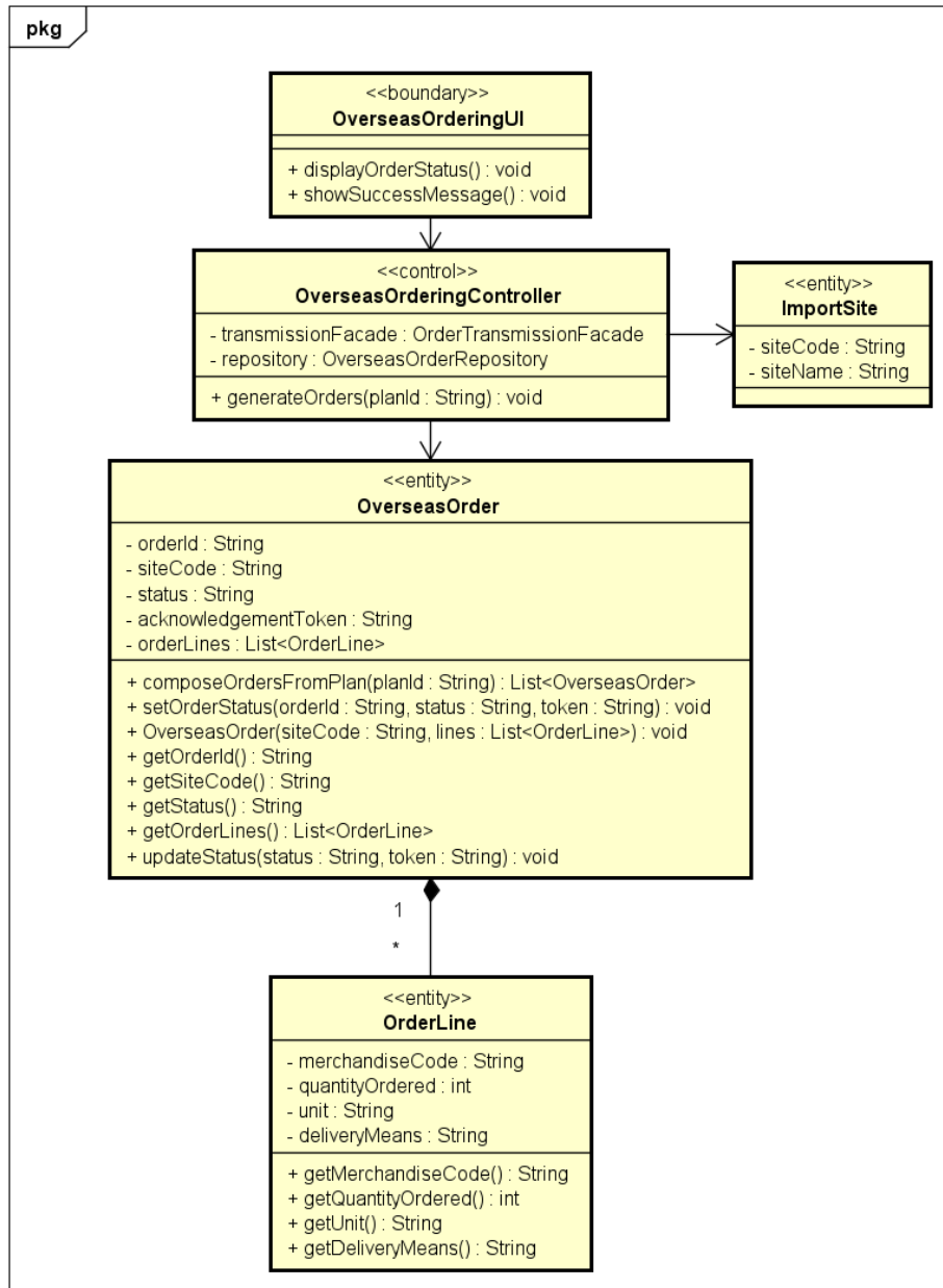
Hình 3.16: Lớp phân tích của PlaceOverseasOrders.
