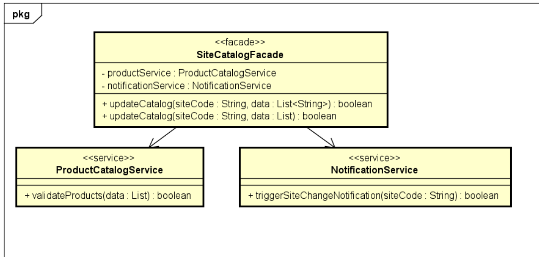
Hình 5.2: Subsystem quản lý danh mục Site cho ManageSiteInformation.
