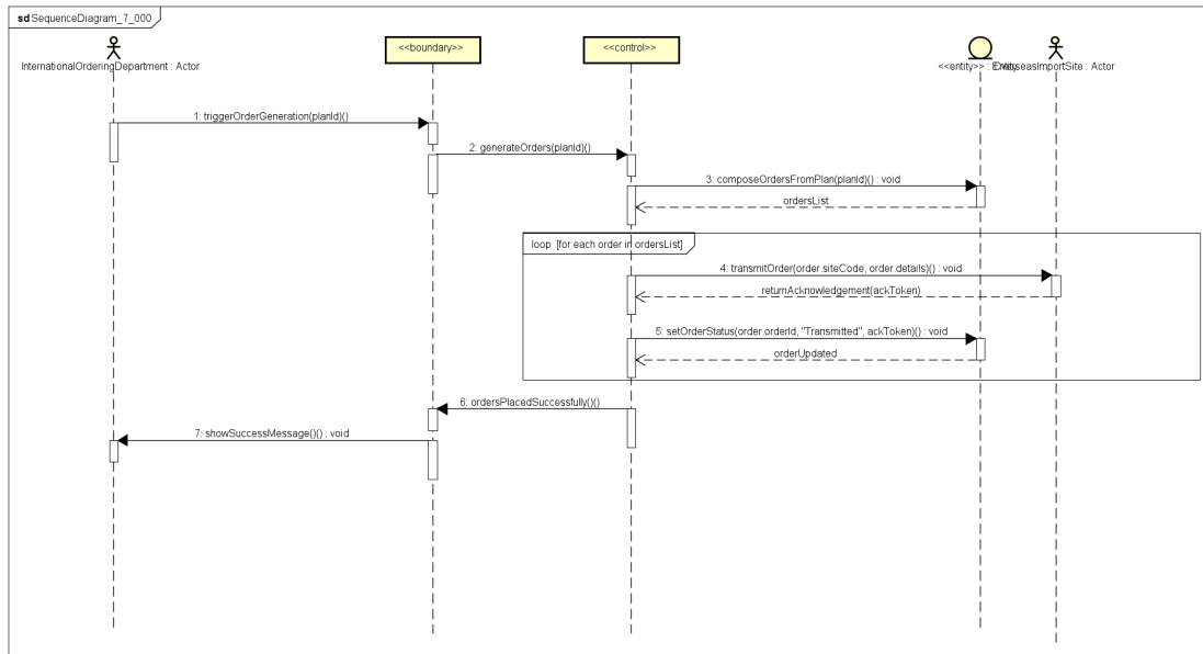
Hình 3.14: Sequence phân tích của PlaceOverseasOrders.
