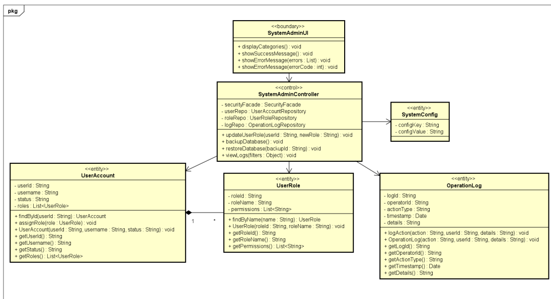
Hình 3.22: Lớp phân tích của ManageSystem.
