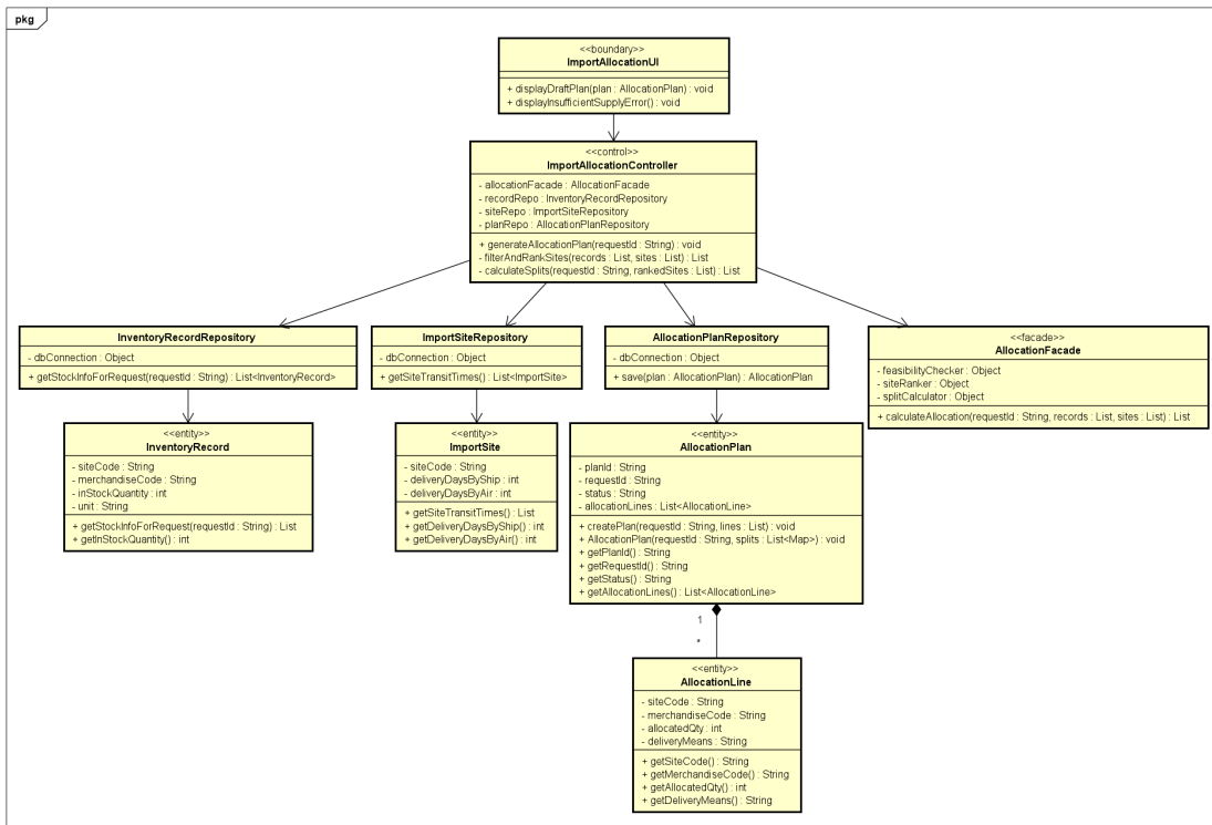
Hình 6.4: Biểu đồ lớp thiết kế của PlanImportAllocation.
