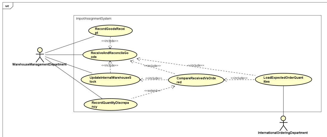
Hình 2.7: Use case phân rã ReceiveAndReconcileGoods.
