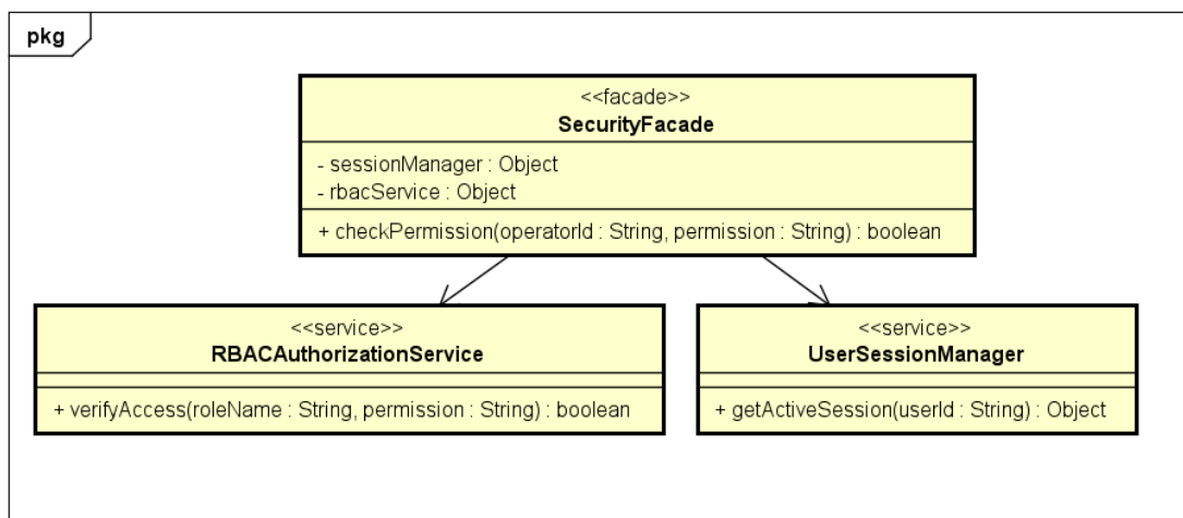
Hình 5.7: Subsystem phân quyền cho ManageSystem .
