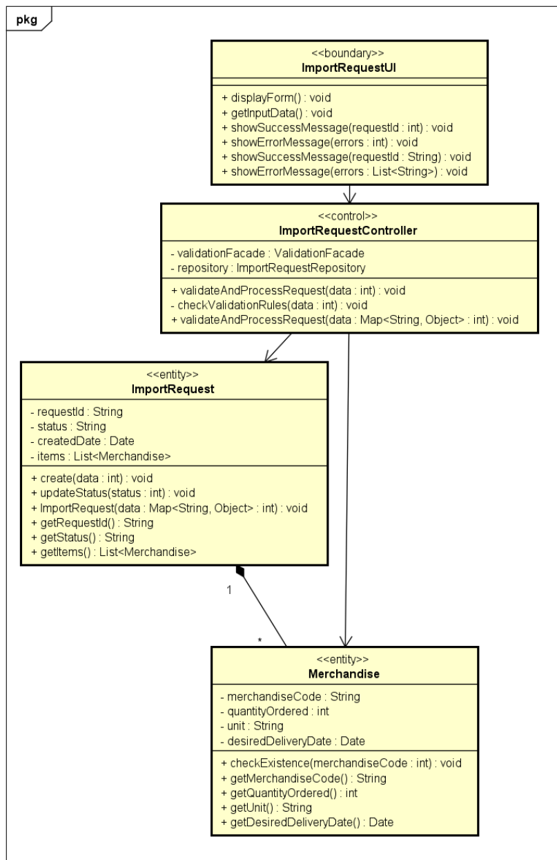
Hình 3.4: Lớp phân tích của ManageImportRequests .
