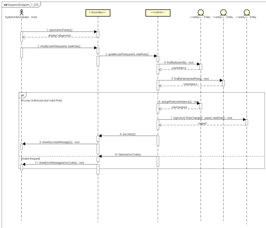
Hình 3.20: Sequence phân tích của ManageSystem.
