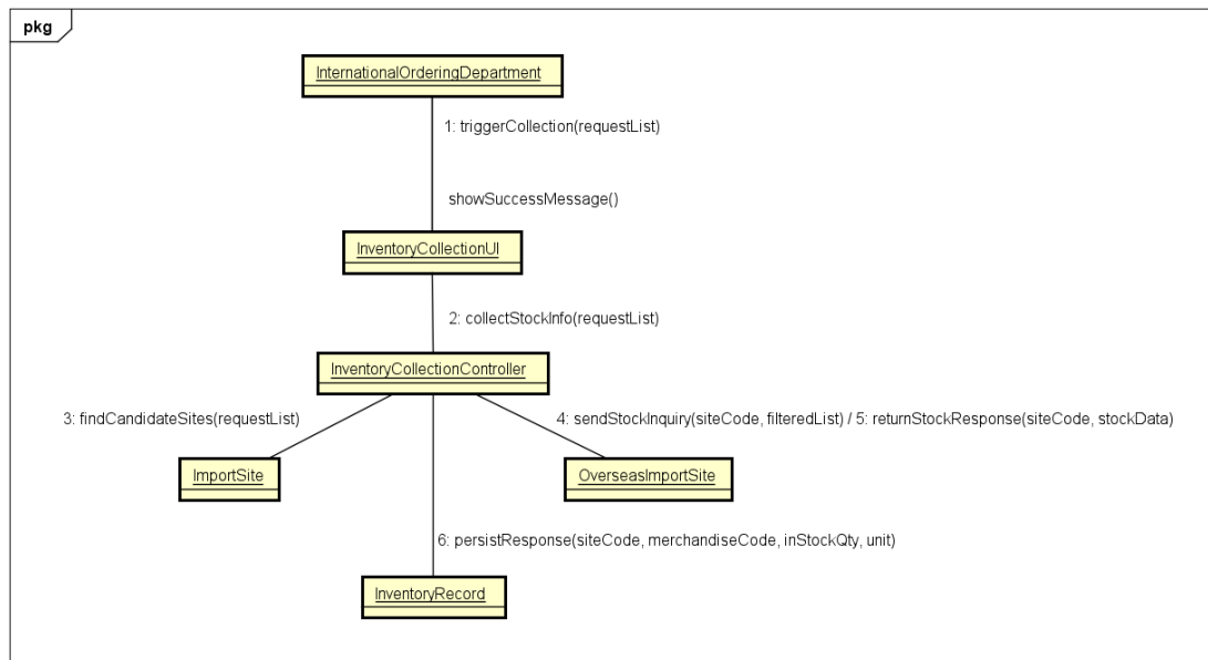
Hình 3.9: Communication phân tích của CollectInventoryData.
