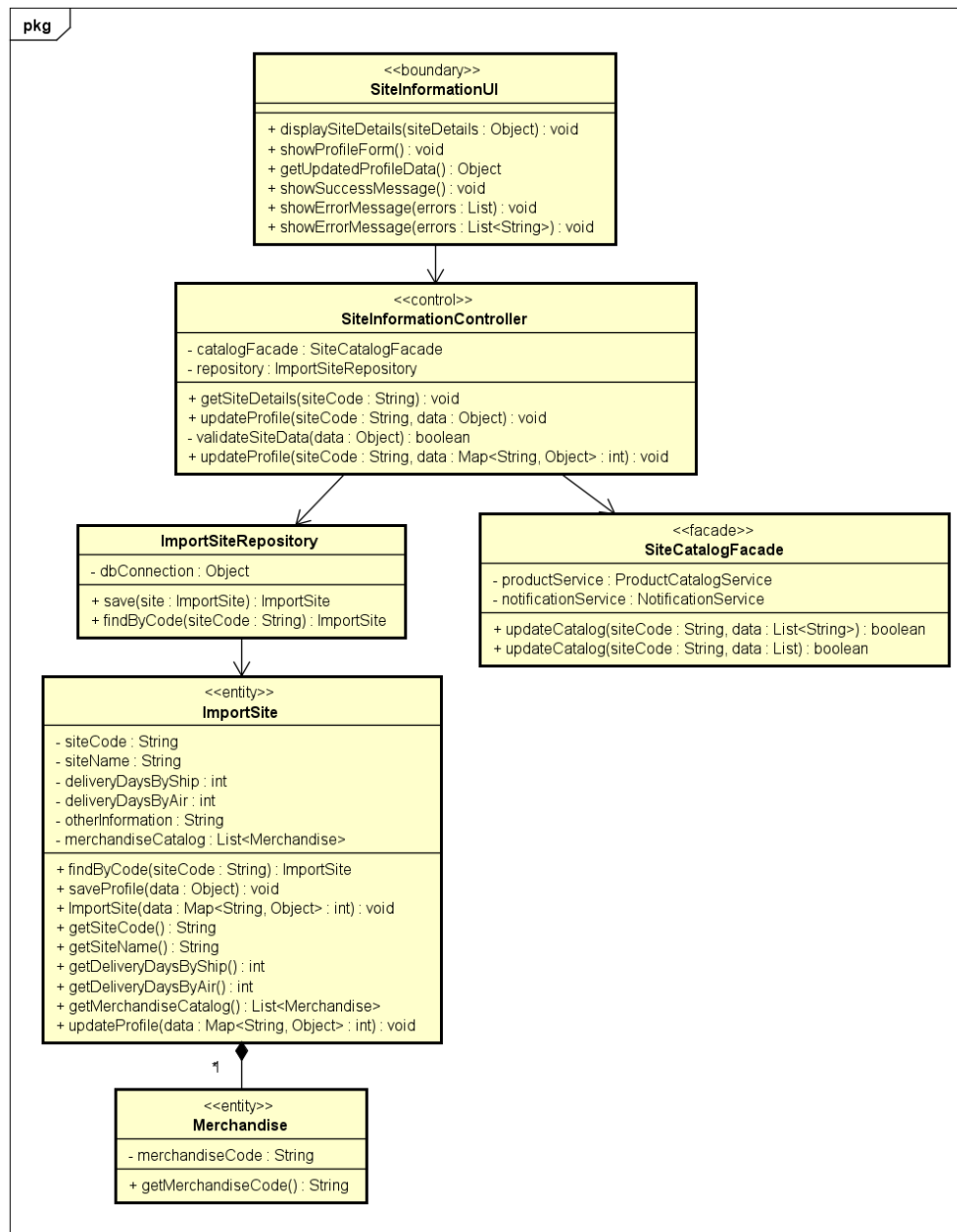
Hình 6.2: Biểu đồ lớp thiết kế của ManageSiteInformation.
