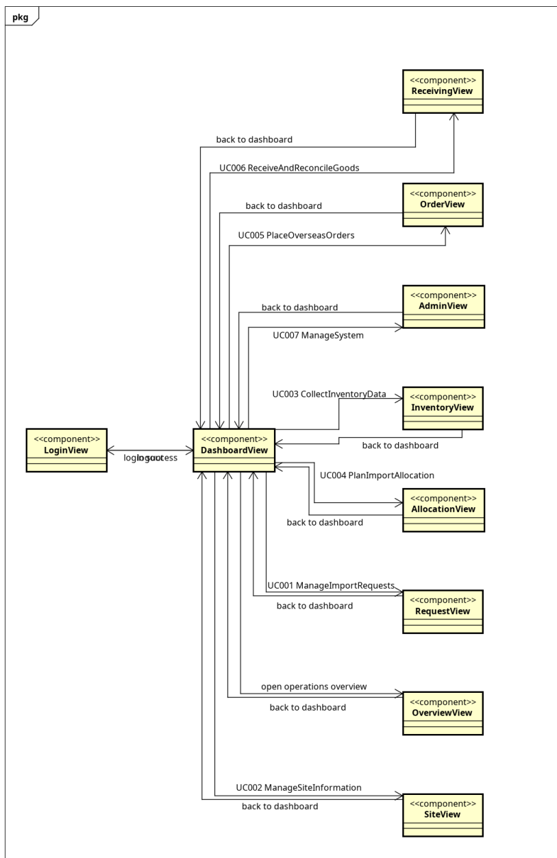
Hình 4.1: Sơ đồ chuyển đổi màn hình tổng quan.
