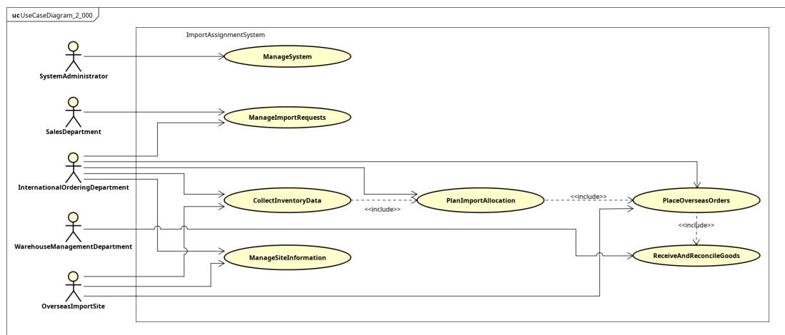
Hình 2.1: Use case tổng quan của hệ thống đặt hàng nhập khẩu.
