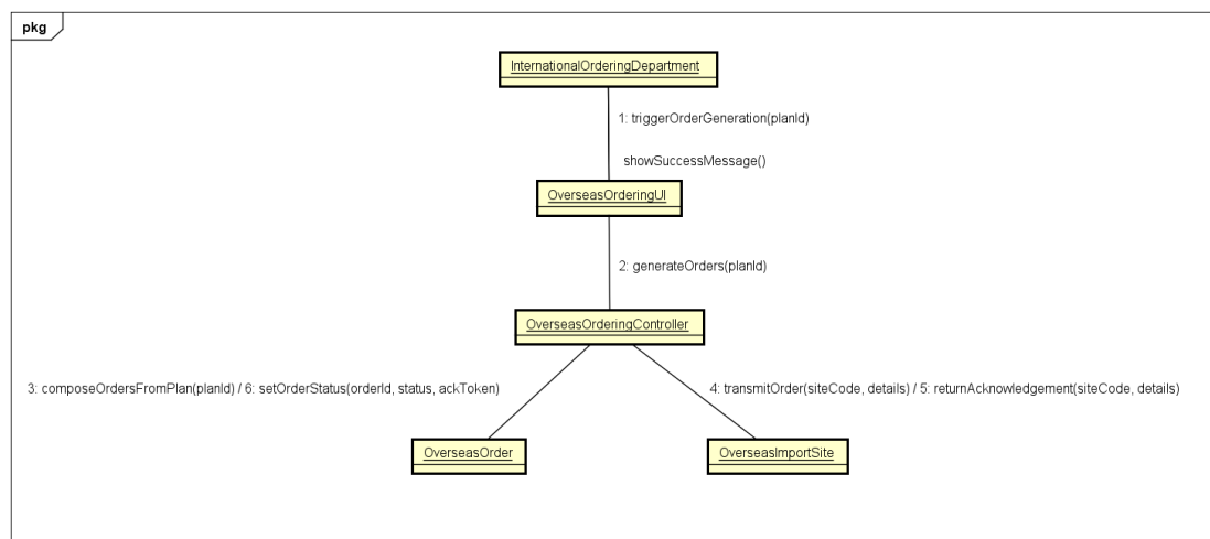
Hình 3.15: Communication phân tích của PlaceOverseasOrders.
