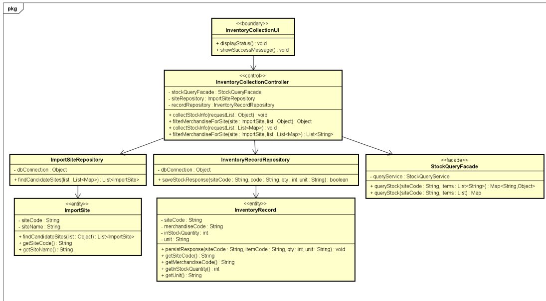
Hình 6.3: Biểu đồ lớp thiết kế của CollectInventoryData.
