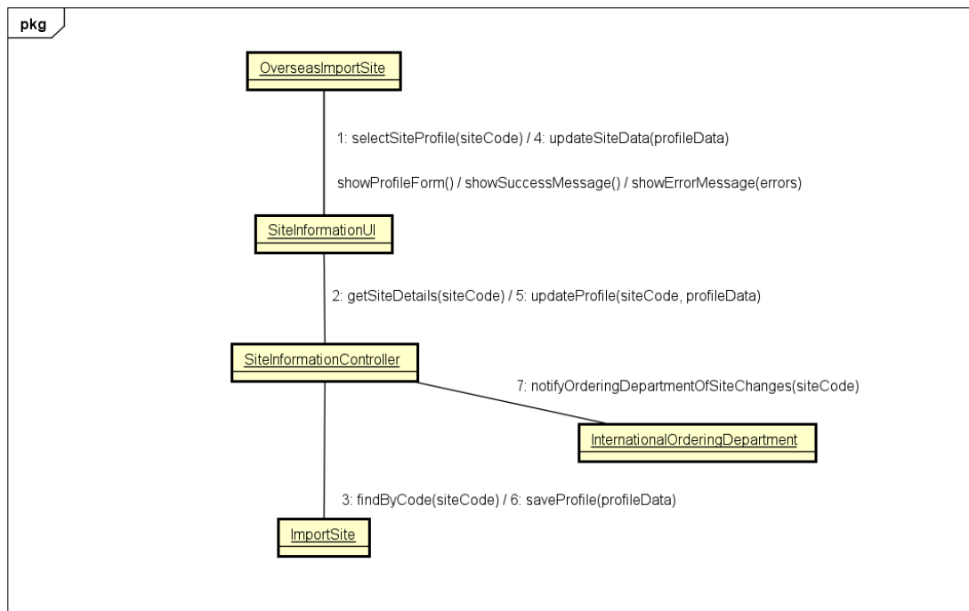
Hình 3.6: Communication phân tích của ManageSiteInformation .
