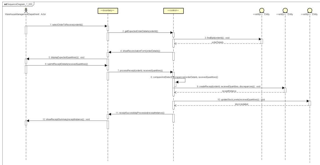
Hình 3.17: Sequence phân tích của ReceiveAndReconcileGoods.
