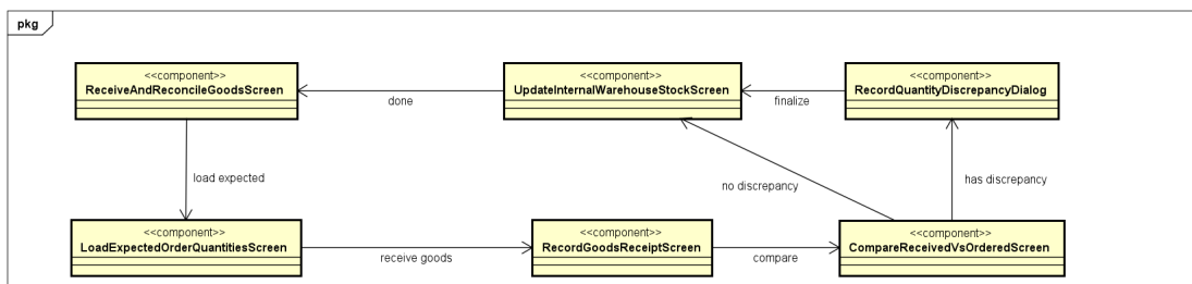
Hình 4.7: Sơ đồ màn hình ReceiveAndReconcileGoods.
