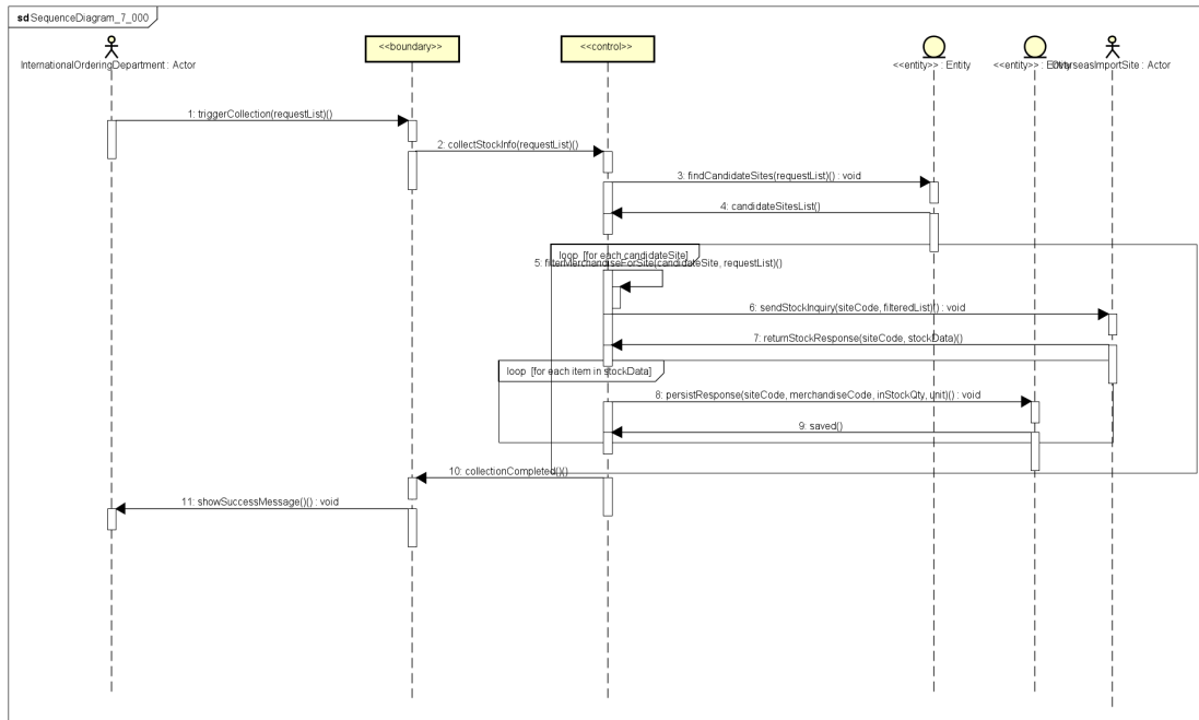
Hình 3.8: Sequence phân tích của CollectInventoryData.
