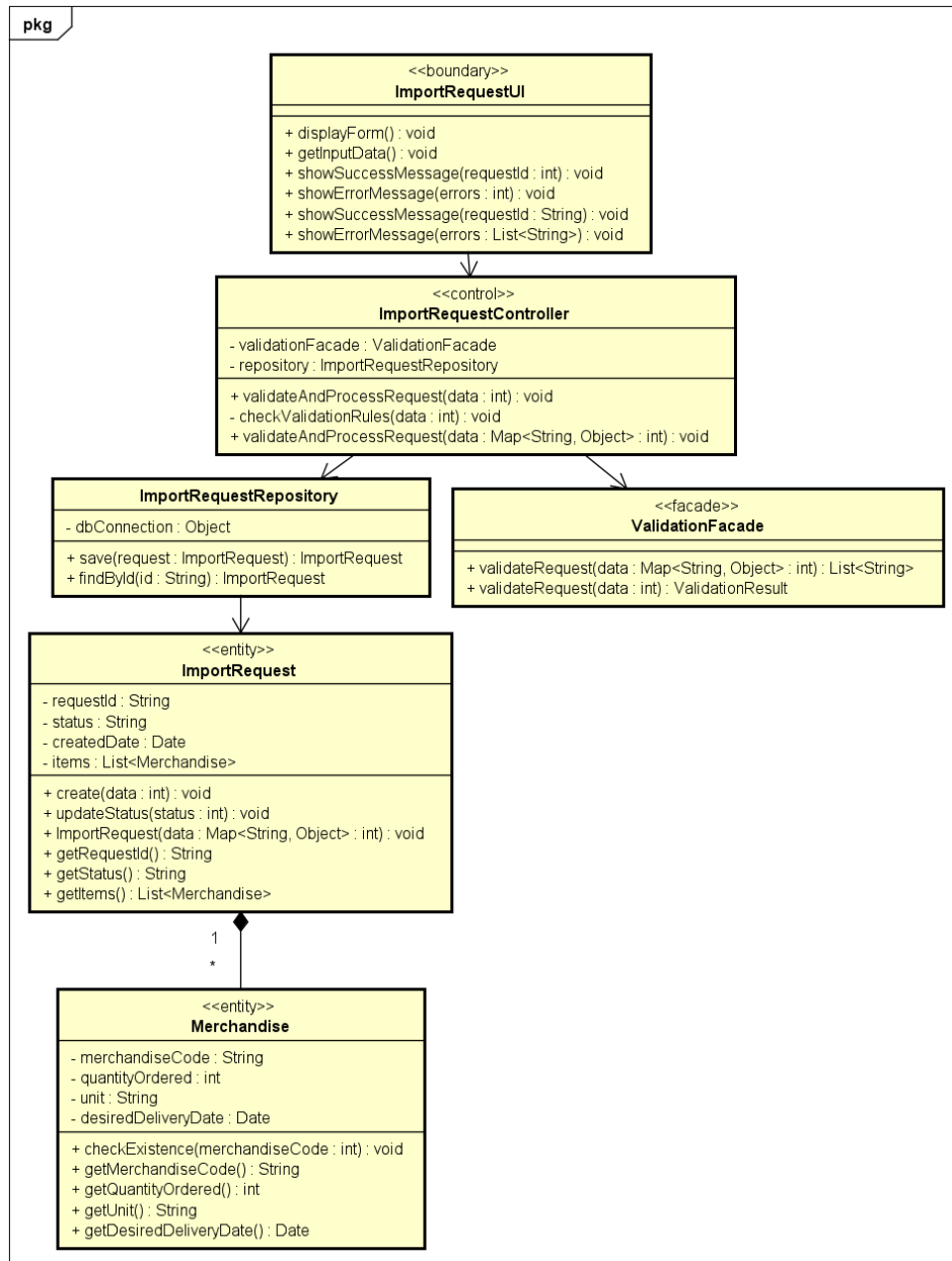
Hình 6.1: Biểu đồ lớp thiết kế của ManageImportRequests.
