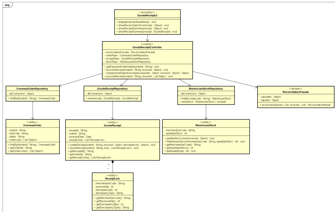
Hình 6.6: Biểu đồ lớp thiết kế của ReceiveAndReconcileGoods.
