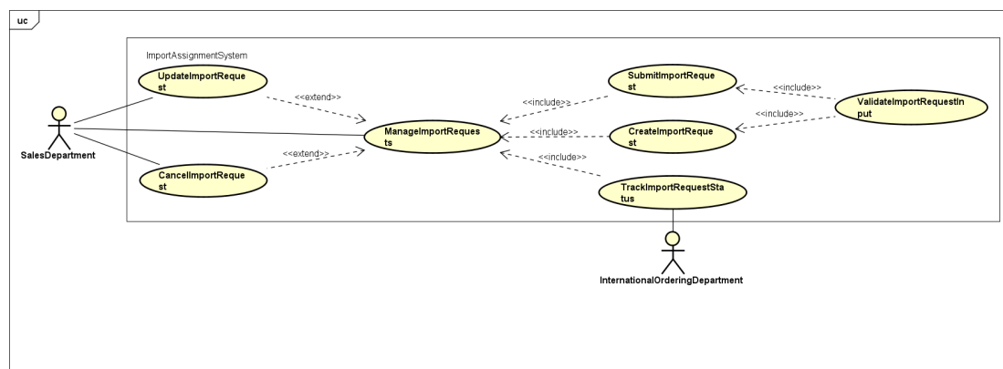
Hình 2.2: Use case phân rã ManageImportRequests.
