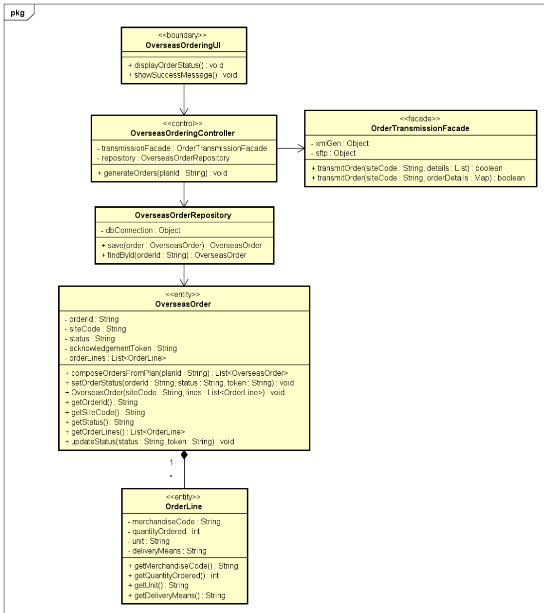
Hình 6.5: Biểu đồ lớp thiết kế của PlaceOverseasOrders.
