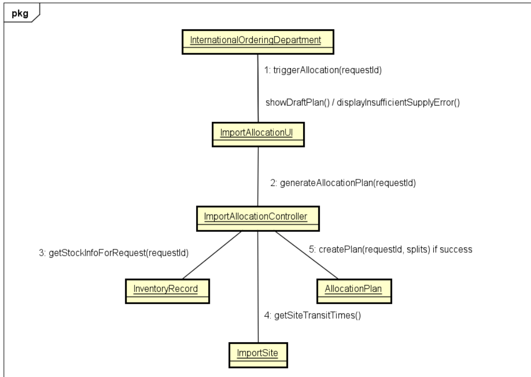
Hình 3.12: Communication phân tích của PlanImportAllocation.
