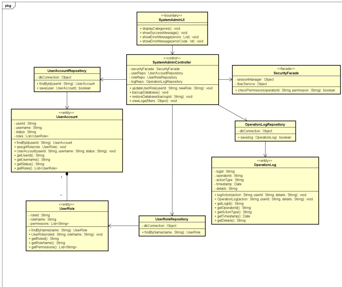
Hình 6.7: Biểu đồ lớp thiết kế của ManageSystem.
