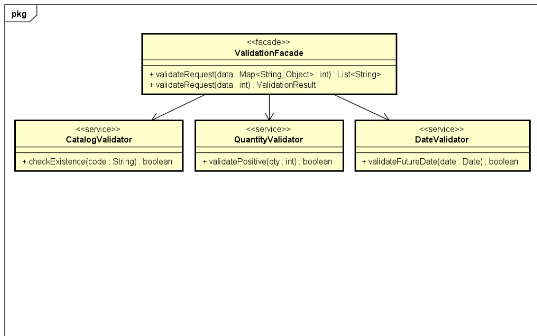
Hình 5.1: Subsystem kiểm tra dữ liệu cho ManageImportRequests.
