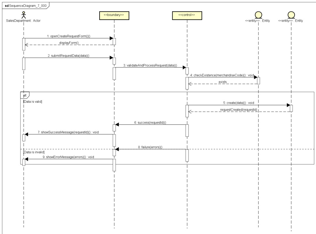
Hình 3.2: Sequence phân tích của ManageImportRequests.
