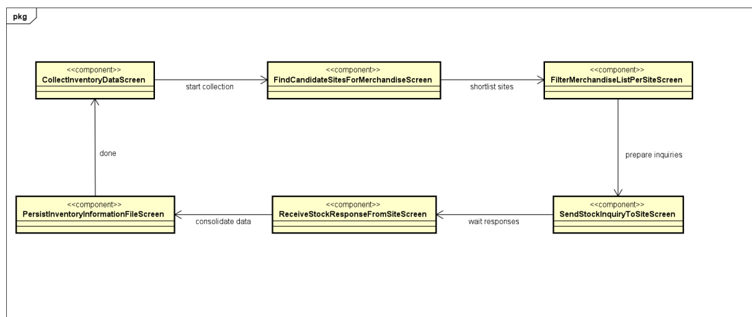
Hình 4.4: Sơ đồ màn hình CollectInventoryData.
