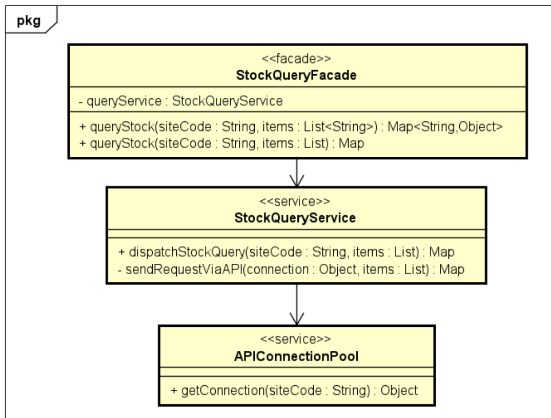
Hình 5.3: Subsystem truy vấn tồn kho cho CollectInventoryData.
