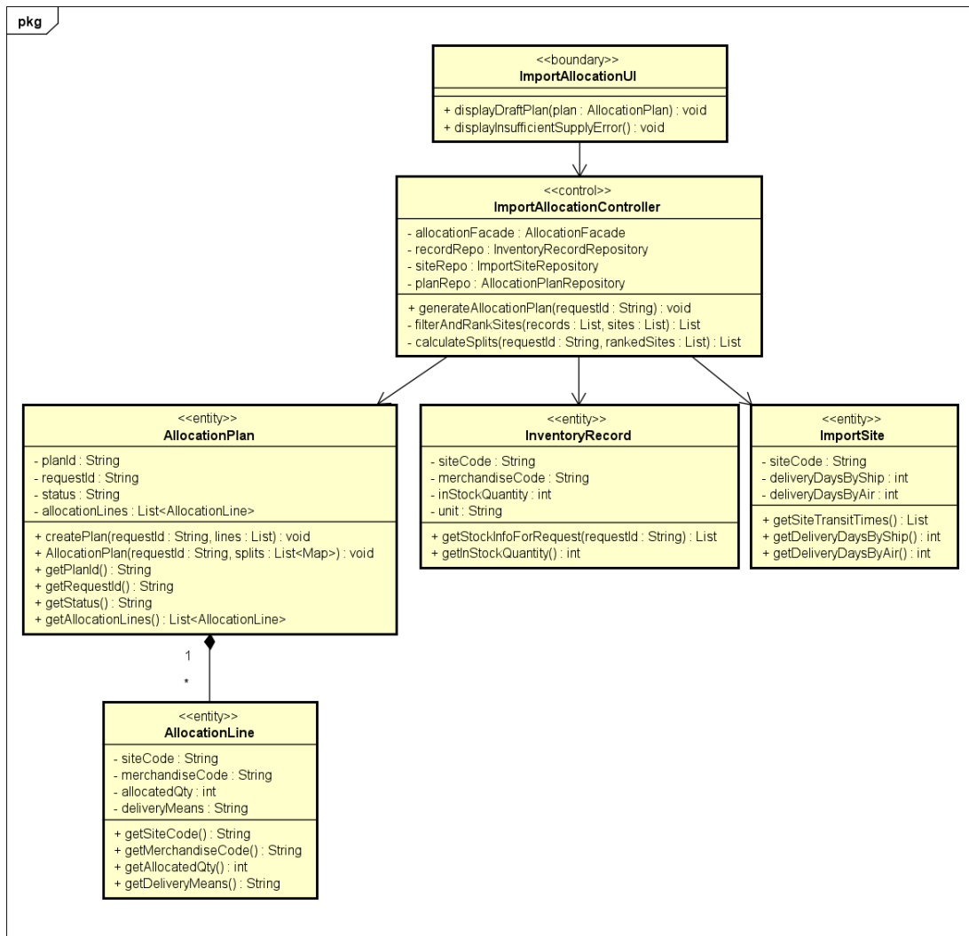
Hình 3.13: Lớp phân tích của PlanImportAllocation.
