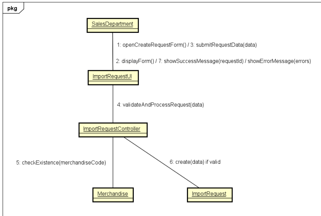
Hình 3.3: Communication phân tích của ManageImportRequests .
