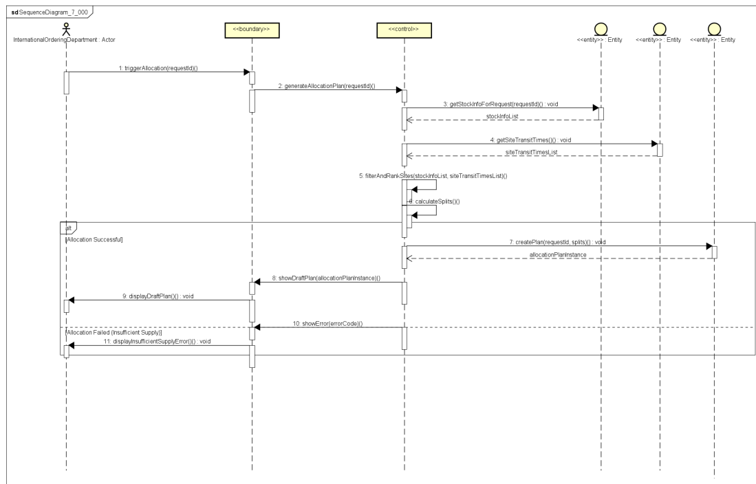
Hình 3.11: Sequence phân tích của PlanImportAllocation.
