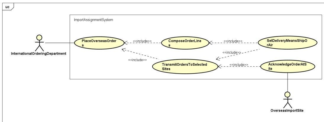
Hình 2.6: Use case phân rã PlaceOverseasOrders.
