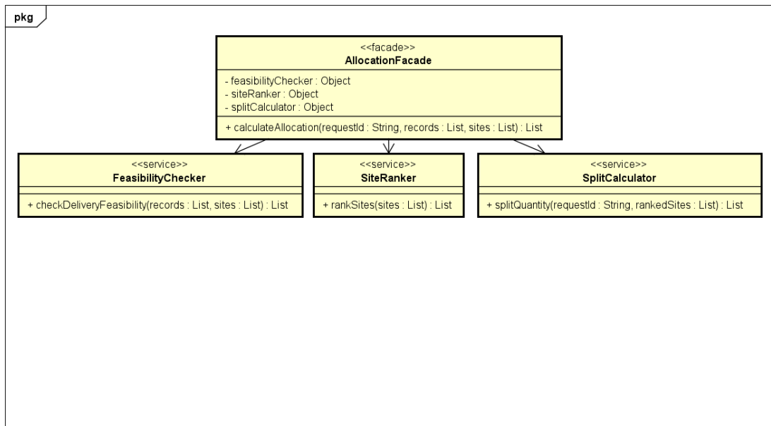
Hình 5.4: Subsystem tính phân bổ cho PlanImportAllocation.
