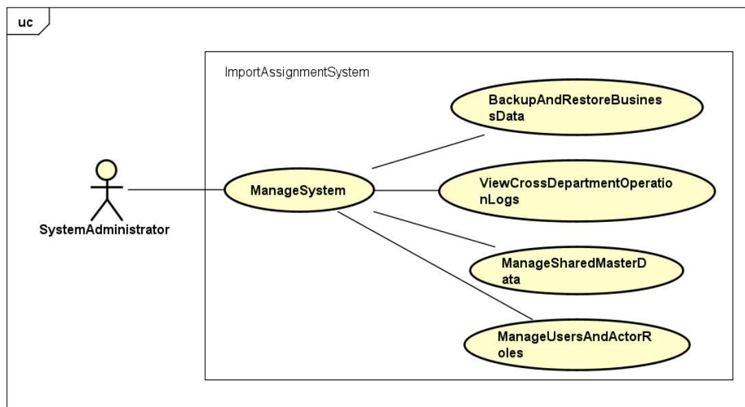
Hình 2.8: Use case phân rã ManageSystem.
