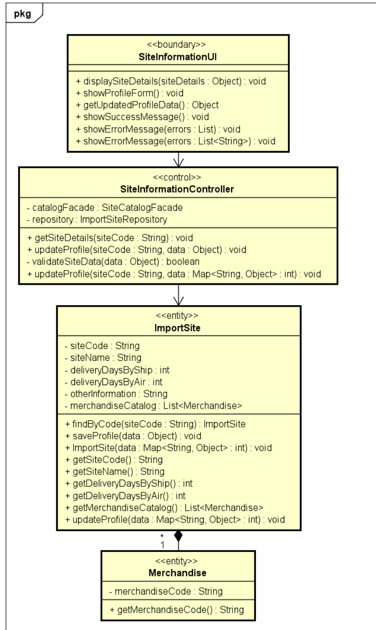
Hình 3.7: Lớp phân tích của ManageSiteInformation.
