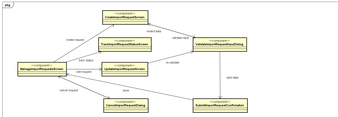
Hình 4.2: Sơ đồ màn hình ManageImportRequests.
