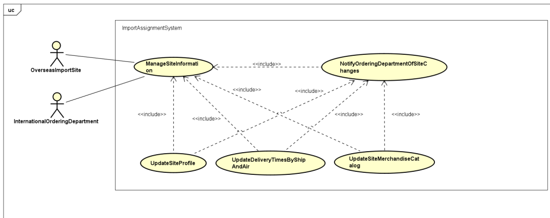
Hình 2.3: Use case phân rã ManageSiteInformation.
