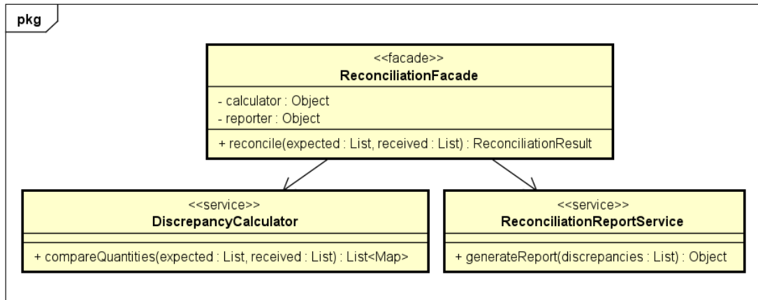
Hình 5.6: Subsystem đối chiếu hàng nhập kho cho ReceiveAndReconcileGoods .
