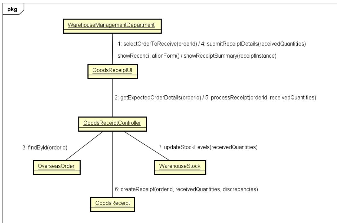
Hình 3.18: Communication phân tích của ReceiveAndReconcileGoods.
