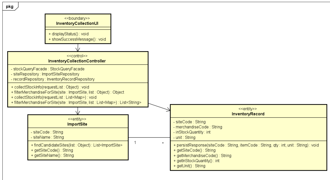
Hình 3.10: Lớp phân tích của CollectInventoryData.
