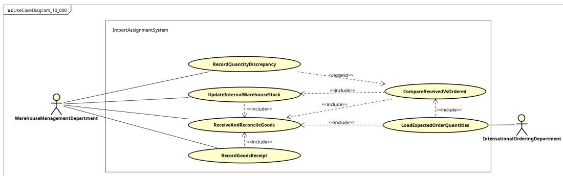
Figure 3.1: Use case phân rã UC006 - ReceiveAndReconcileGoods
