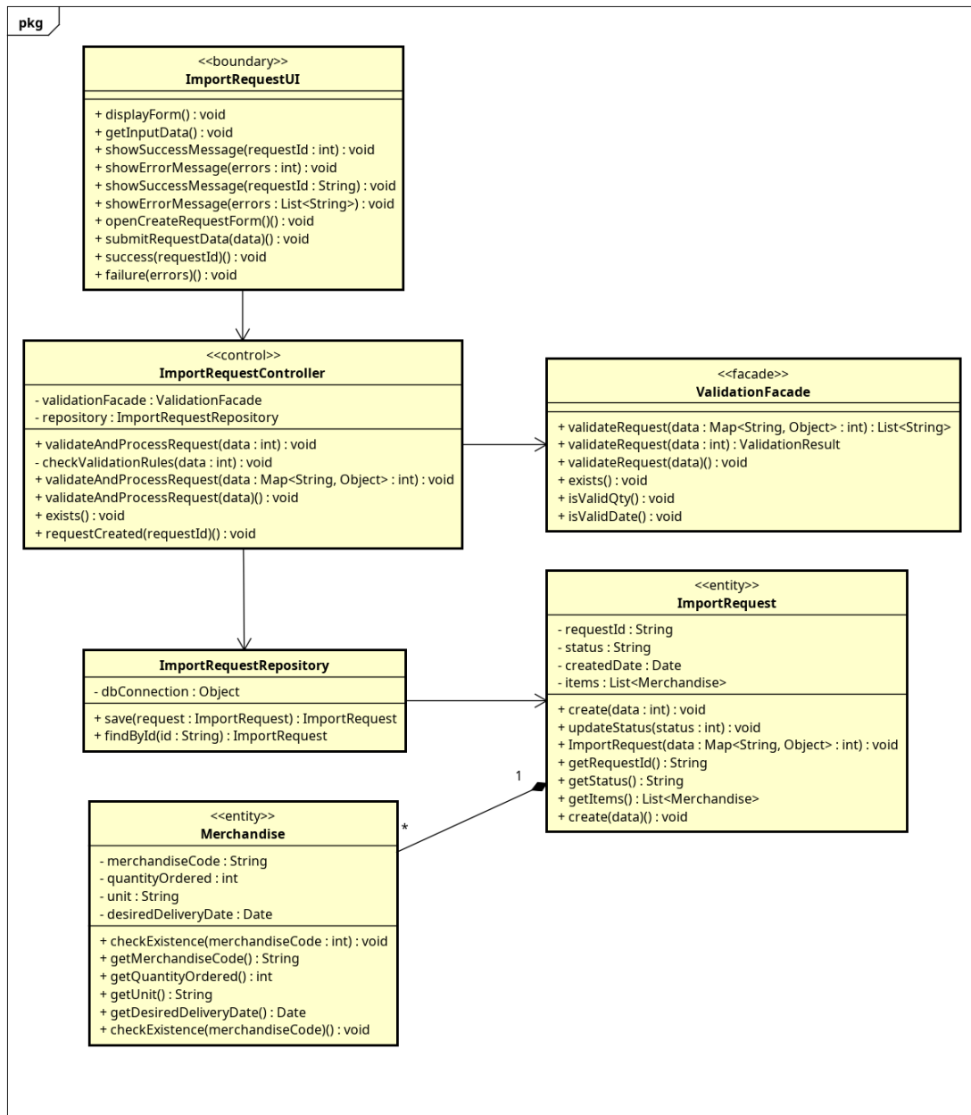
Figure 3.3: Class diagram mức thiết kế UC001 - ManageImportRequests
