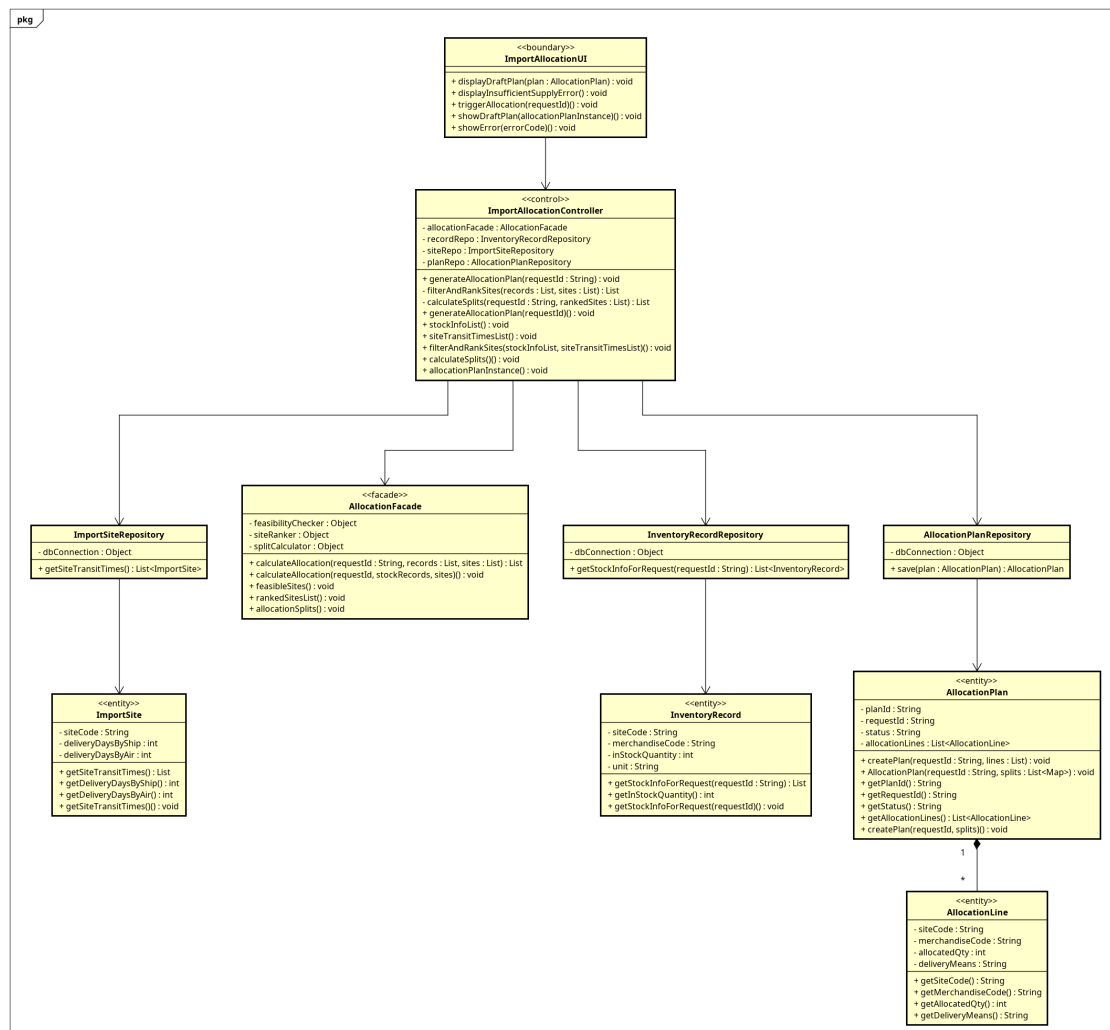
Figure 3.12: Class diagram mức thiết kế UC004 - PlanImportAllocation
