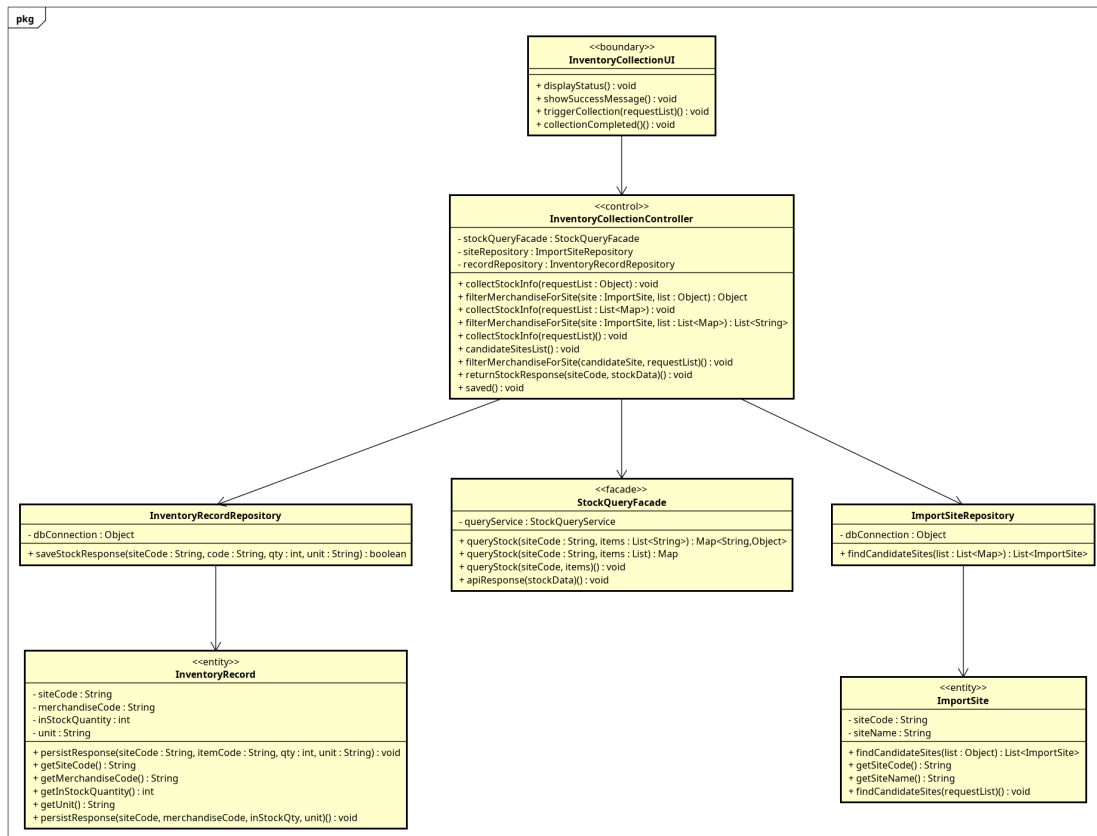
Figure 3.9: Class diagram mức thiết kế UC003 - CollectInventoryData
