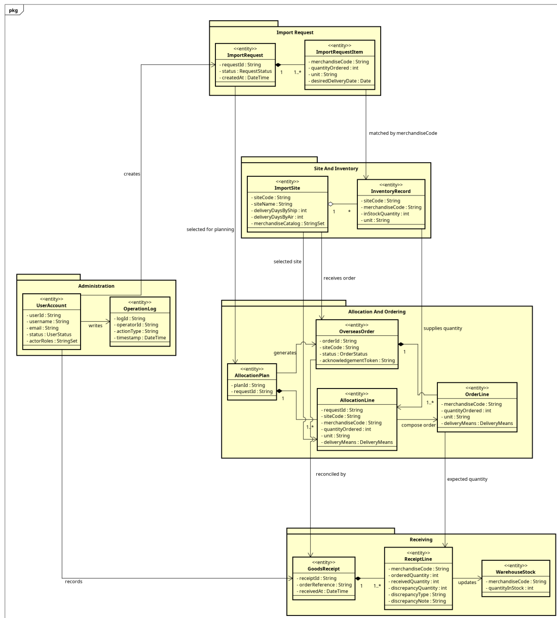
Figure 3.1: Kiến trúc lớp tổng quan
