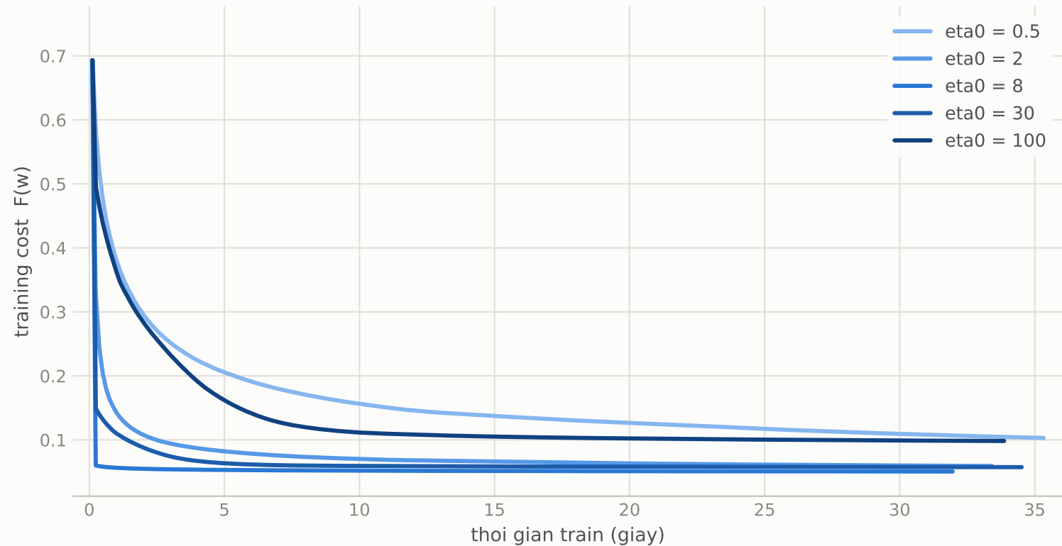
Subgradient (Lasso): quet eta0
