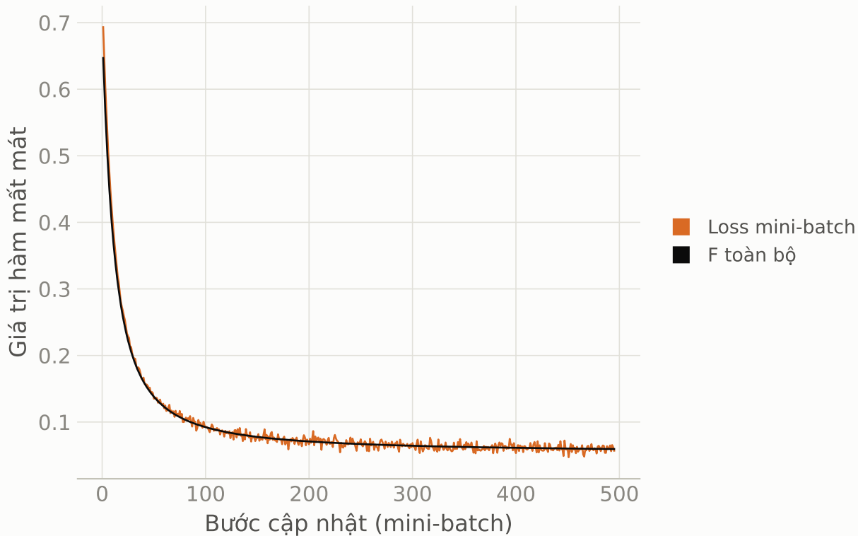
SGD: mini-batch và toàn bộ
