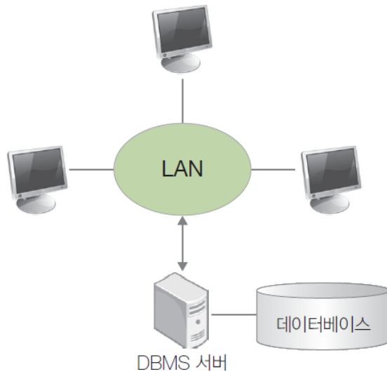
그림 1-12 데이터베이스 시스템
