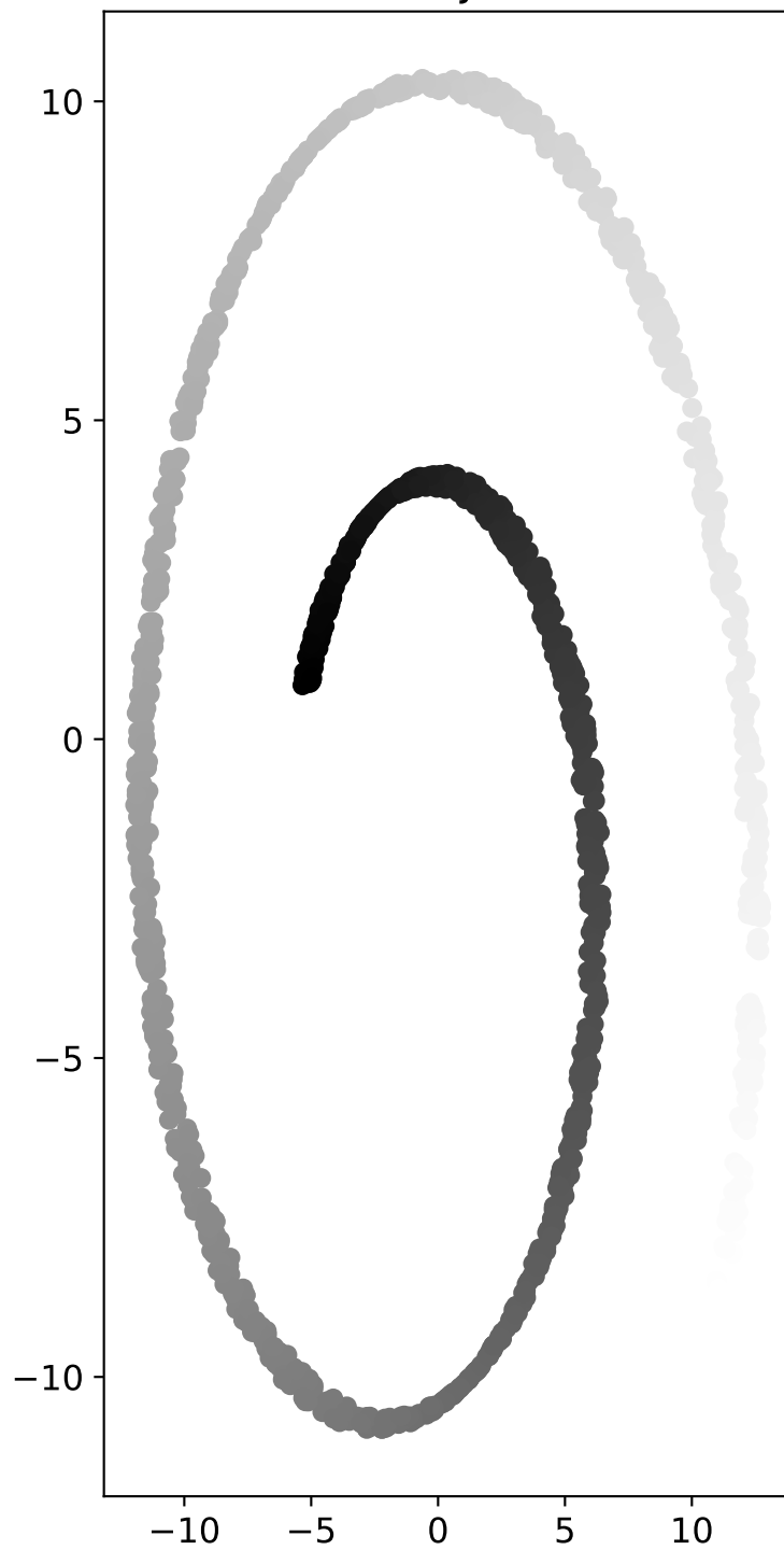
PCA Projection
