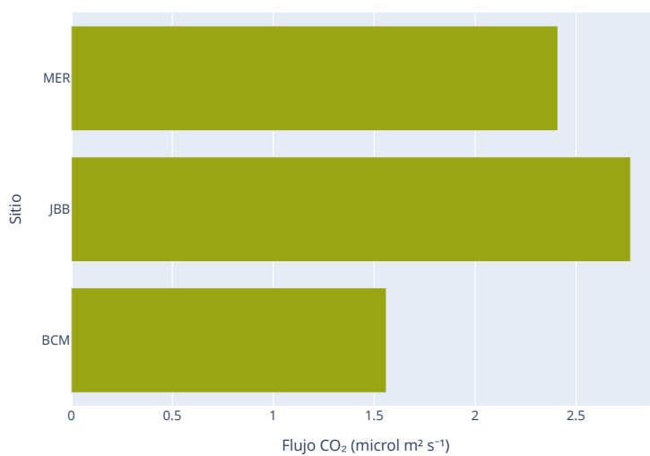
Figura 33: Flujo de gas carbónico en el suelo.
