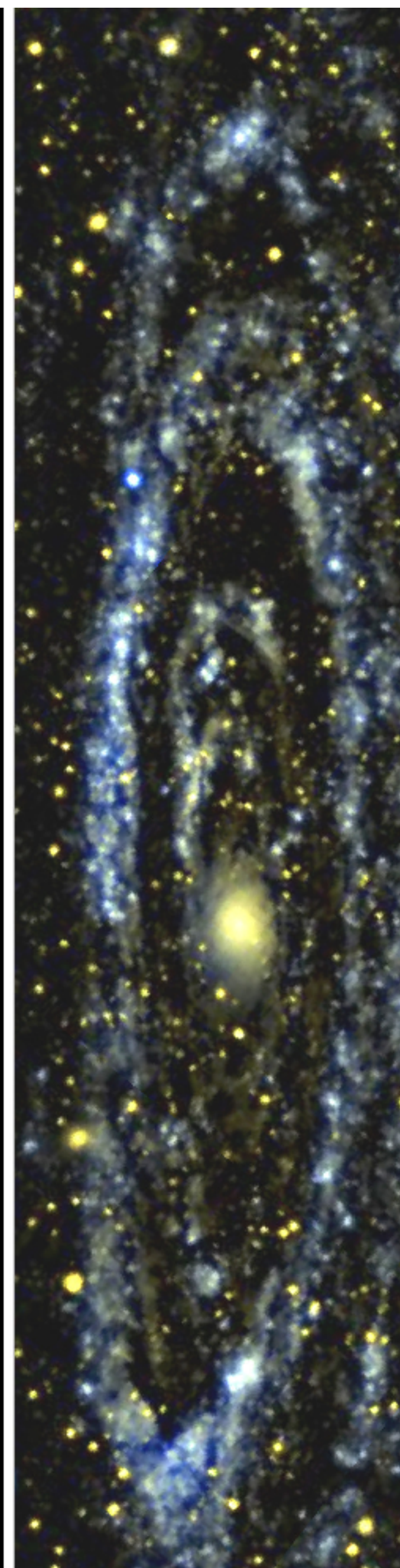
GALEX UV
