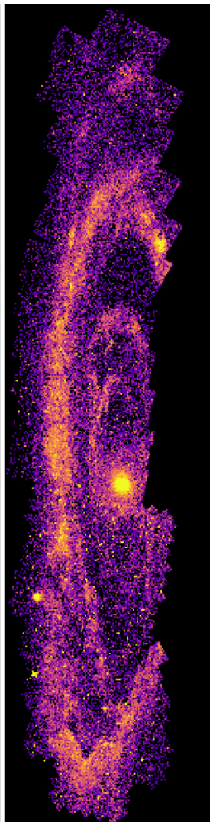
HeB
