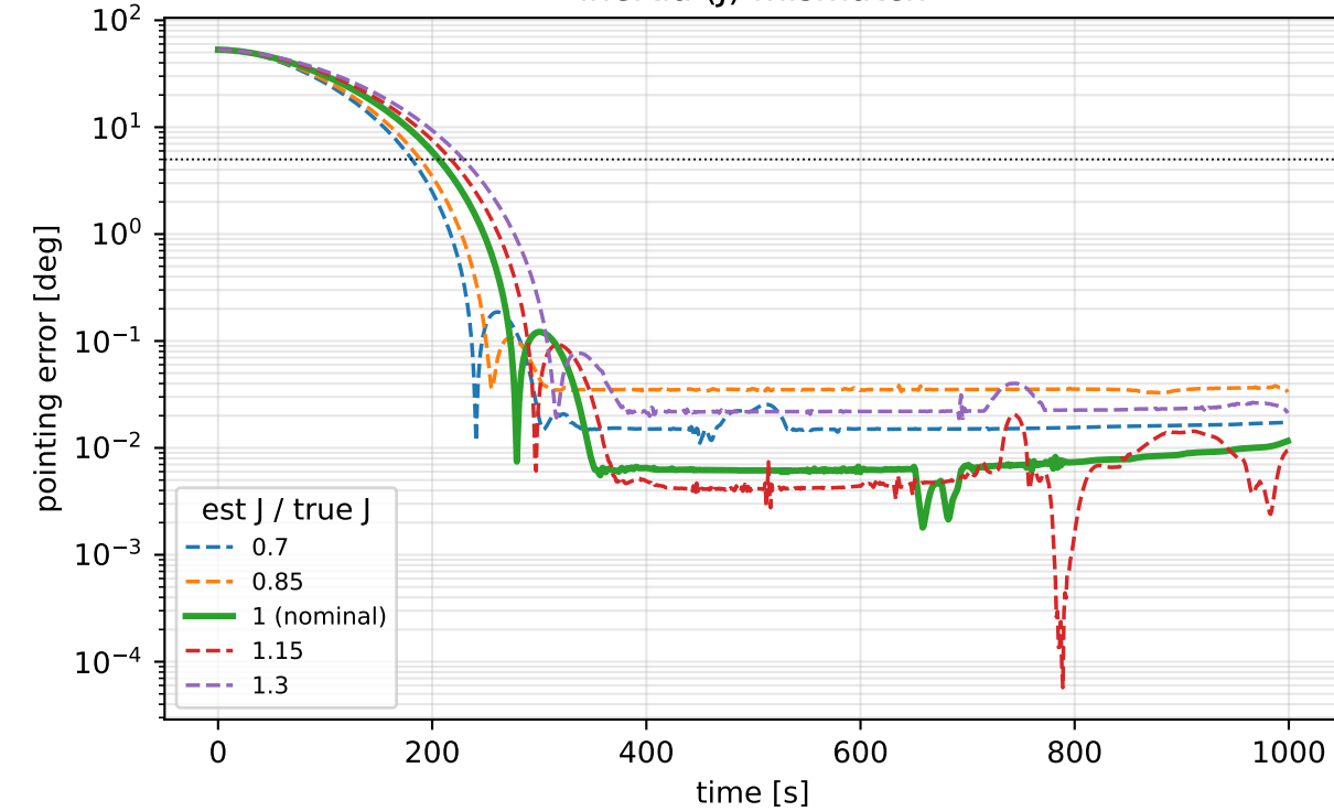
inertia (J) mismatch
