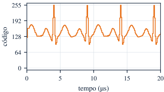
(e) arbitrária, ECG inicial, 100 kHz
