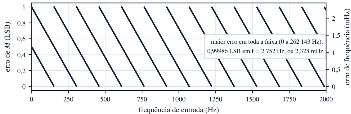
(b) erro de truncamento de M , de 0 a 2 kHz
