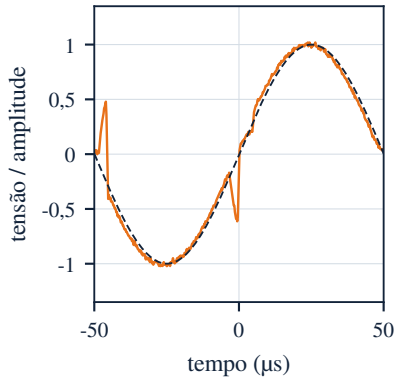
(a) saída, 10 kHz
