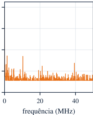
(b) 100 Hz, até 50 MHz
