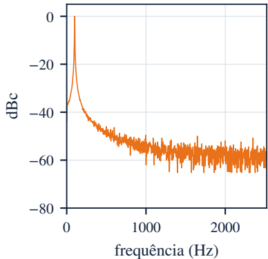
(a) 100 Hz, até 2,5 kHz
