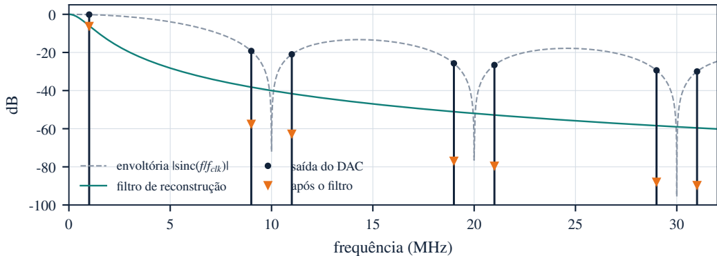
(b) saída do DAC para f_{out} = 1 \text{ MHz} e f_{clk} = 10 \text{ MHz} : imagens e filtro
