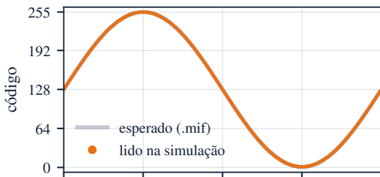
(a) seno (ROM)
