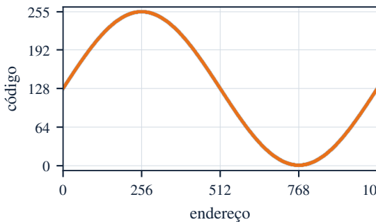
(e) seno com escrita simultânea na RAM
