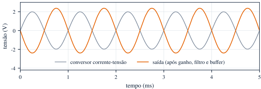
(a) seno de 1 kHz: cinco períodos
