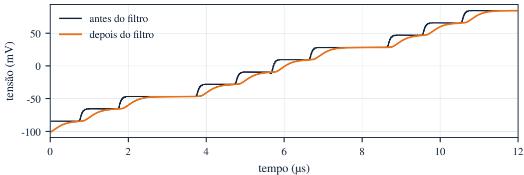
(b) detalhe de uma subida: degraus de um código e o sinal filtrado
