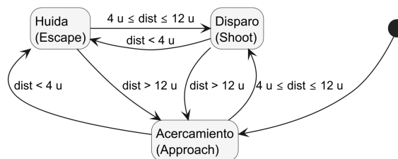
Figura 4.8: Diagrama de la FSM del SlimeGreen. Elaboración propia.
