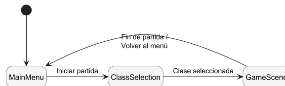
Figura 3.2: Diagrama del flujo de escenas. Elaboración propia.
