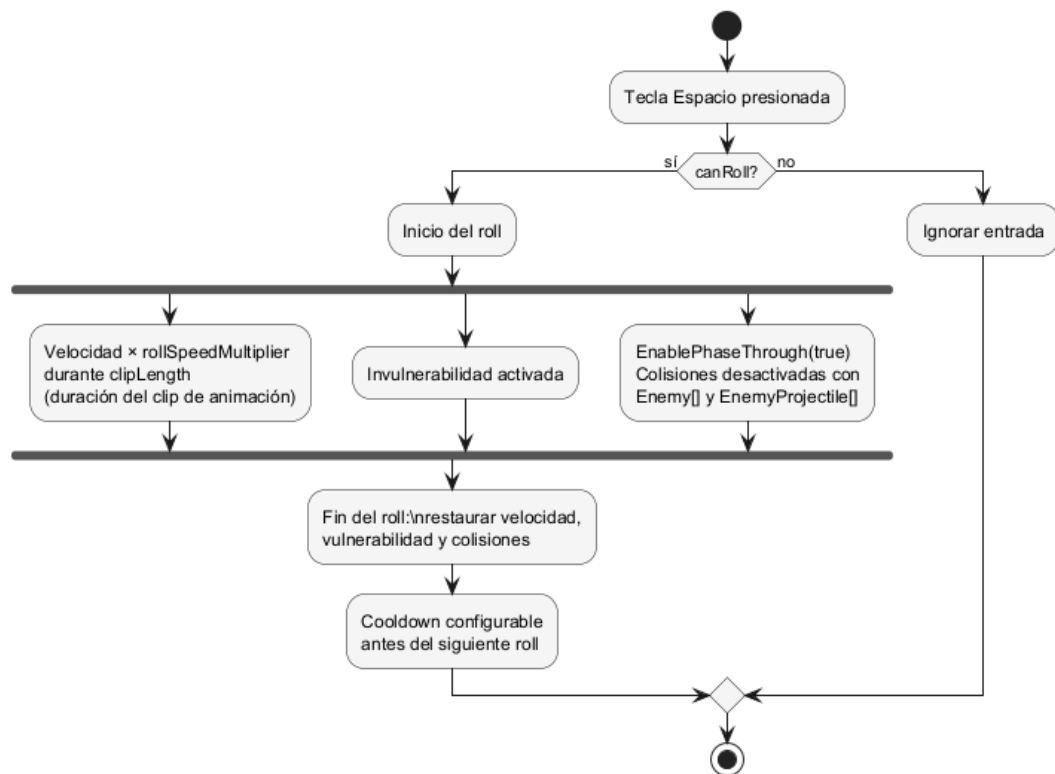
Figura 4.6: Diagrama del funcionamiento de la esquivada. Elaboración propia.
