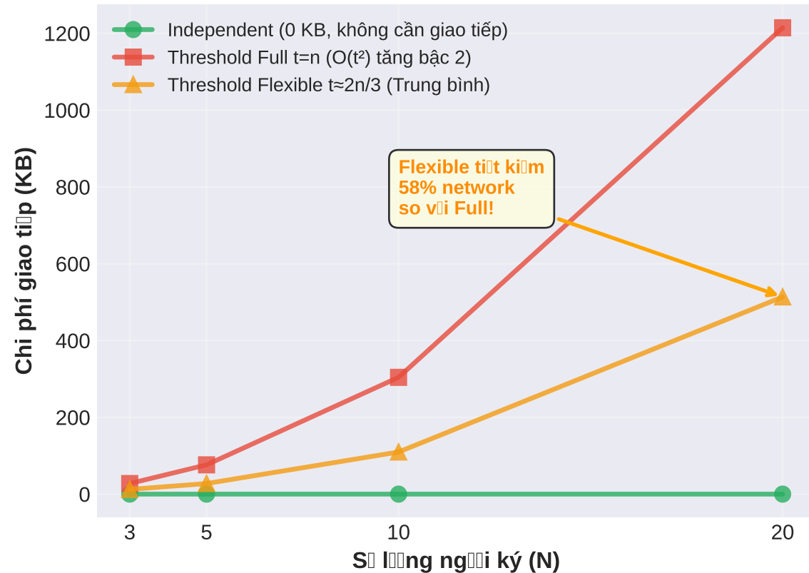
Biểu đồ 3: The Communication Cost Trade-off phí chấp nhận ( O(t^2) network)
