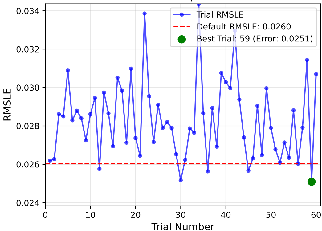
HPO Error per Trial
