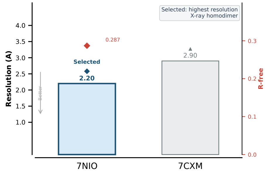
NSP13-Helicase
