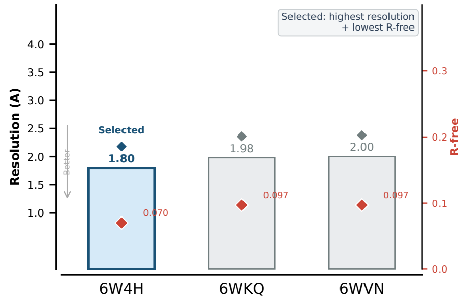
NSP10-NSP16
