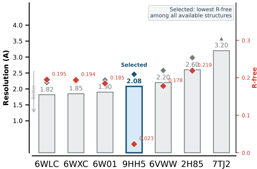
NSP15
