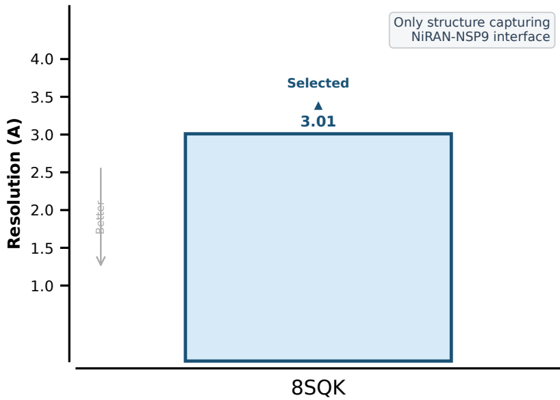
NSP9-NSP12
