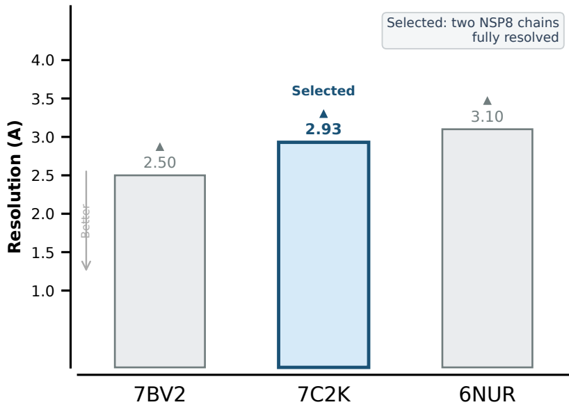
NSP12-NSP8
