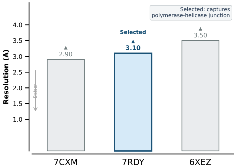
NSP12-NSP13
