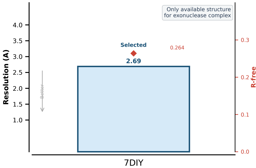
NSP10-NSP14
