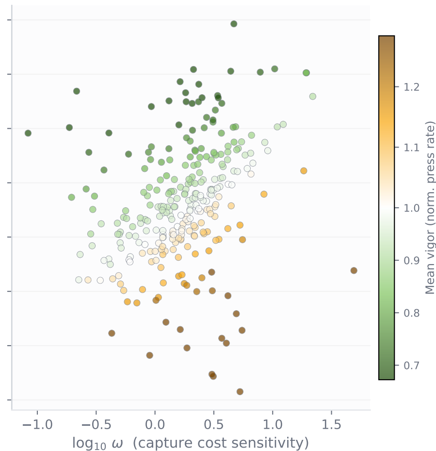
Confirmatory (N=281)
