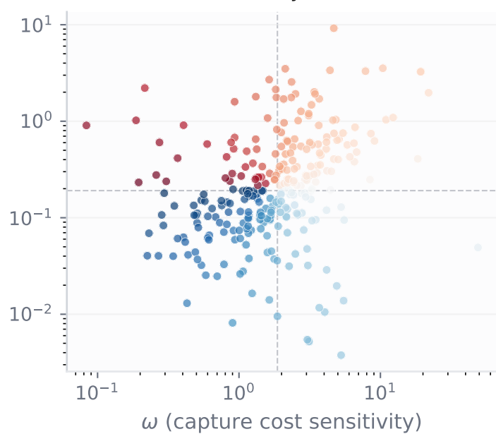
Confirmatory (N=281)
