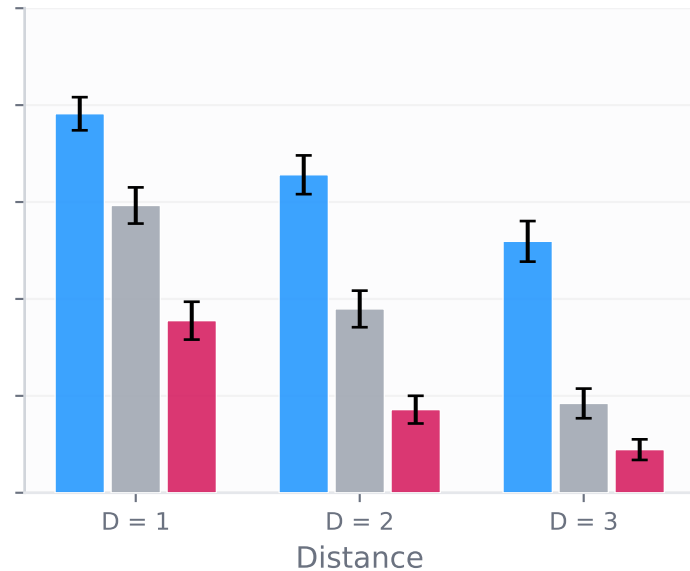
Confirmatory (N=281)
