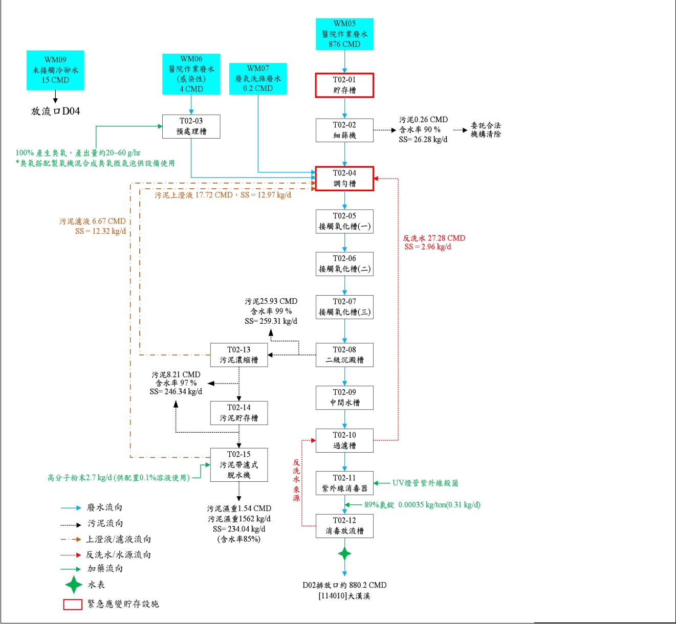
亞東醫院第二院區 廢水流程圖 設計水量以88%計算
