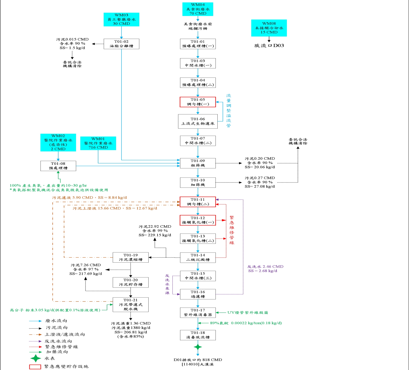
亞東醫院第一院區 廢水流程圖 設計水量以88%計算
