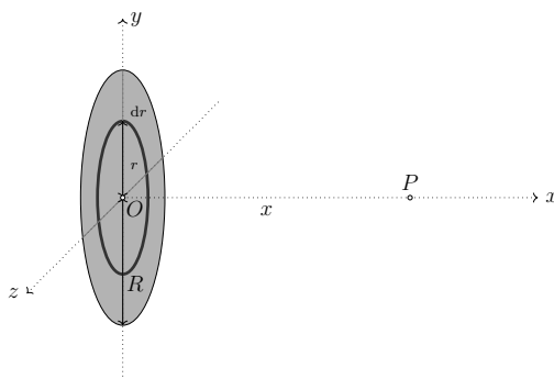
图 8.6: 均匀带电圆盘的电场
