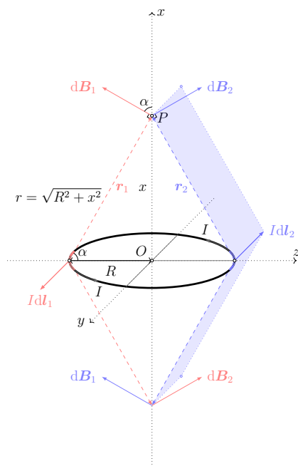
图10.6: 载流圆线圈的磁场
