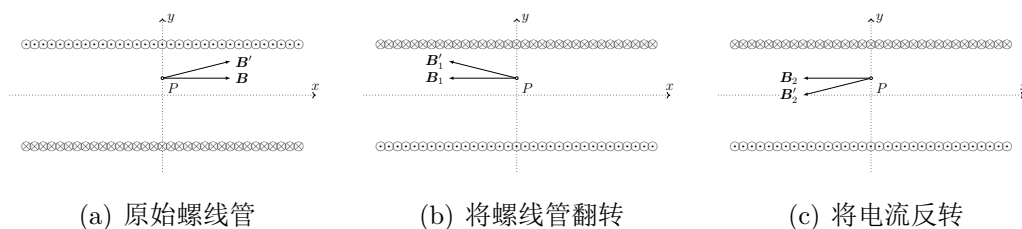
图 10.14: 证明螺旋管内外的磁场方向
