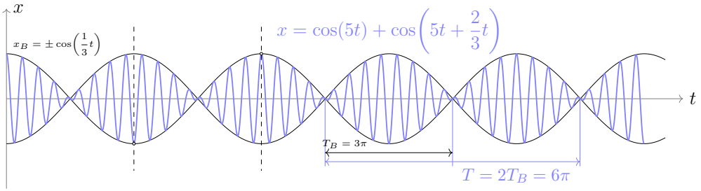
(b) 拍频与合振动频率不同的情况
