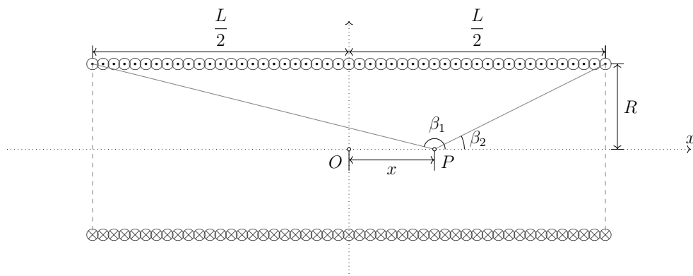
图 10.10: 载流螺线管的中心坐标
