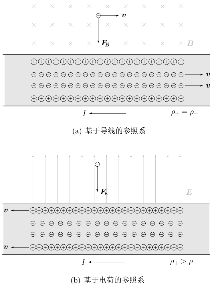
图 10.13: 磁场与电场的统一性
