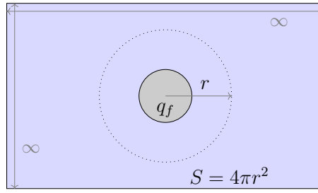
图 9.21: 浸在无限大均匀电介质中的导体球
