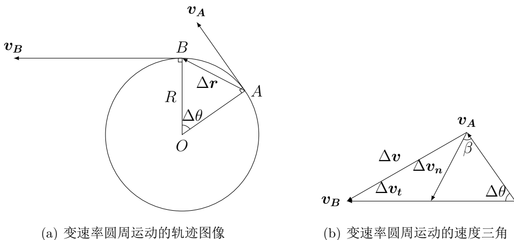
图 1.2: 变速率圆周运动
