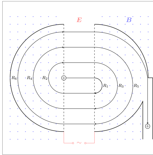
图 10.20: 回旋加速器
