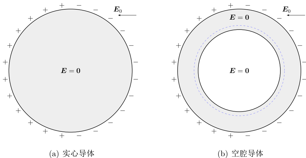
图 9.3: 空腔导体的电荷分布与电场分布
