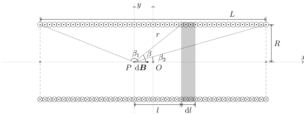
图 10.9: 载流螺线管的磁场
