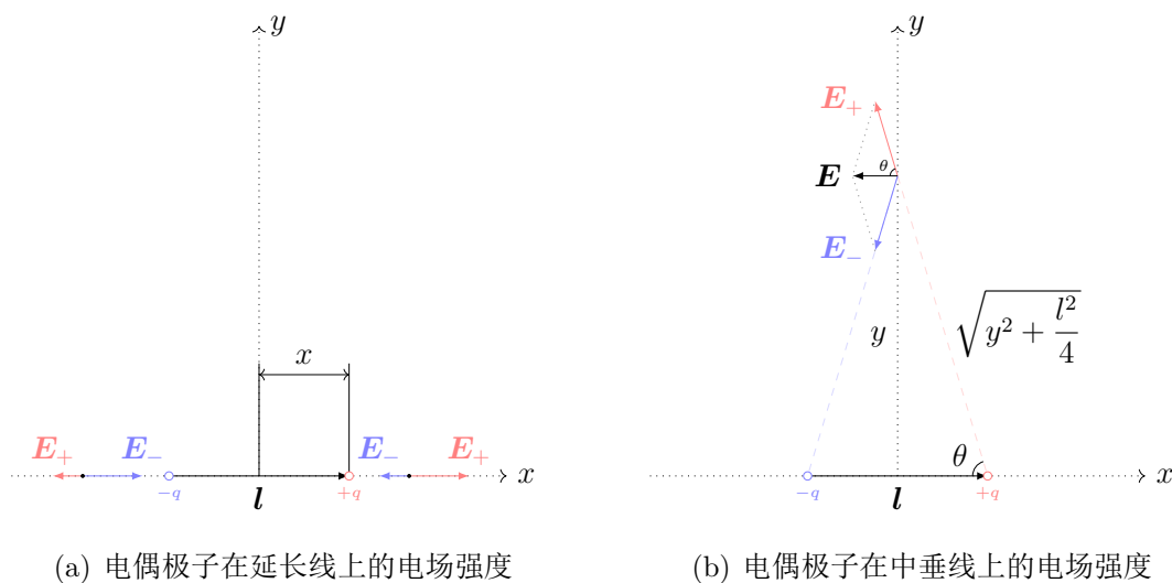
图 8.3: 电偶极子的电场强度
