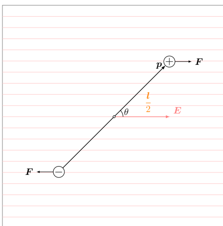
图 8.12: 静电场中的电偶极子
