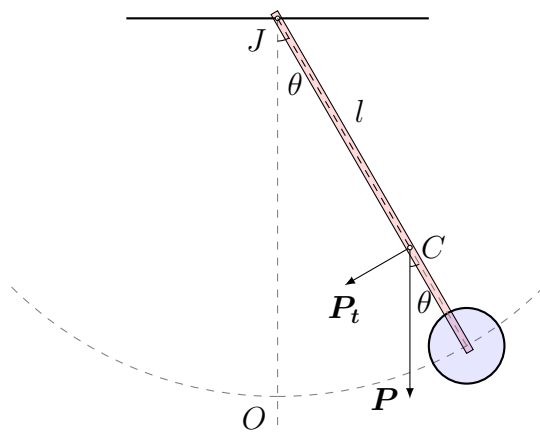
图 6.4: 复摆的示意图
