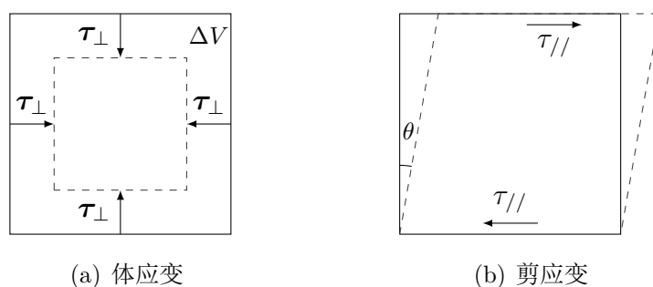
图 7.4: 体应变与剪应变
