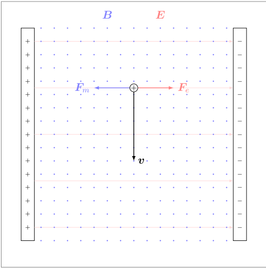
图 10.21: 速度选择器
