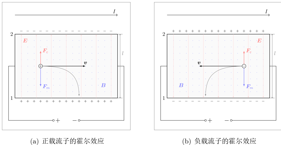
图 10.24: 霍尔效应
