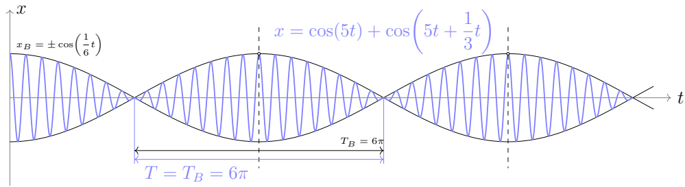
(a) 拍频与合振动频率相同的情况
