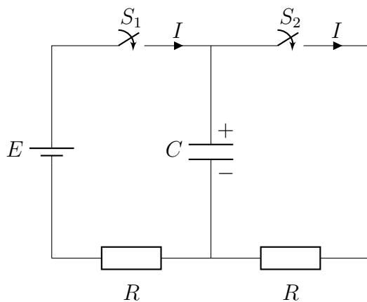
图 9.8: RC 电路
