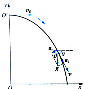
图 20: 例题 L1-3 图
