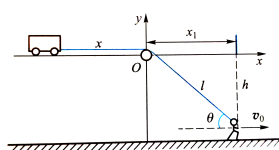
图 19: 例题 L1-2 图
