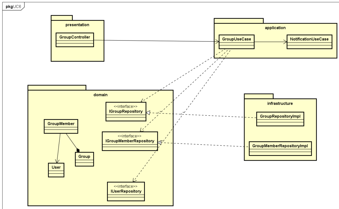
Hình 48: Biểu đồ gói chi tiết cho UC6: Quản lý nhóm
