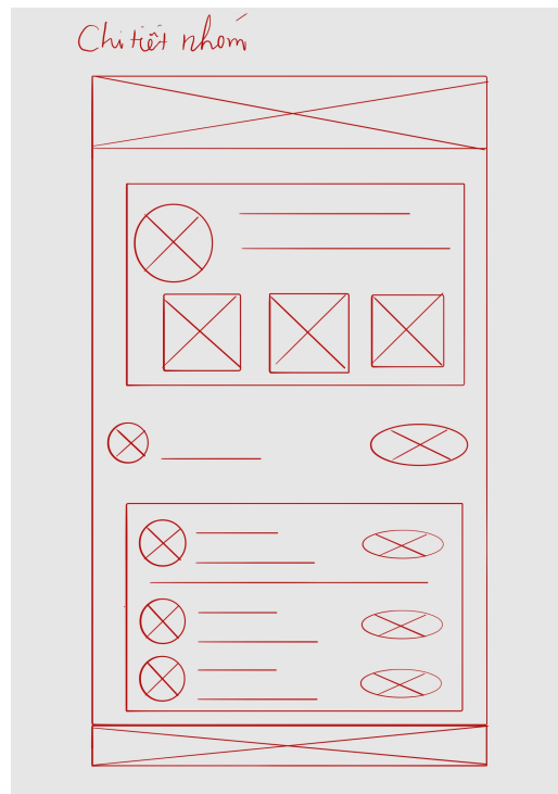
Hình 15: Thiết kế giao diện cho UC6: Quản lý nhóm - chi tiết nhóm
