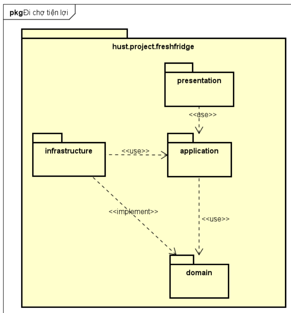
Hình 42: Sơ đồ phân lớp các gói (Package Diagram) theo Clean Architecture
