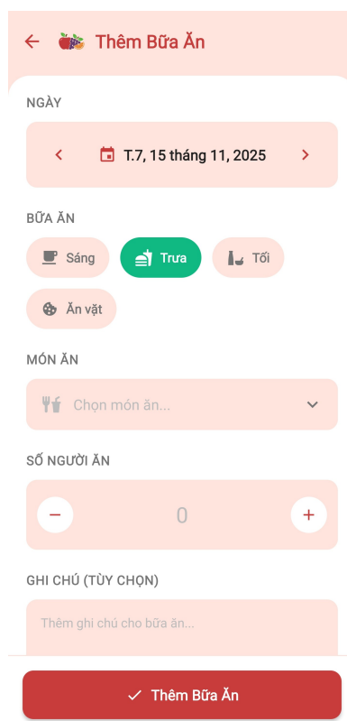
Hình 26: Thiết kế giao diện quản lý dự định bữa ăn - 2
