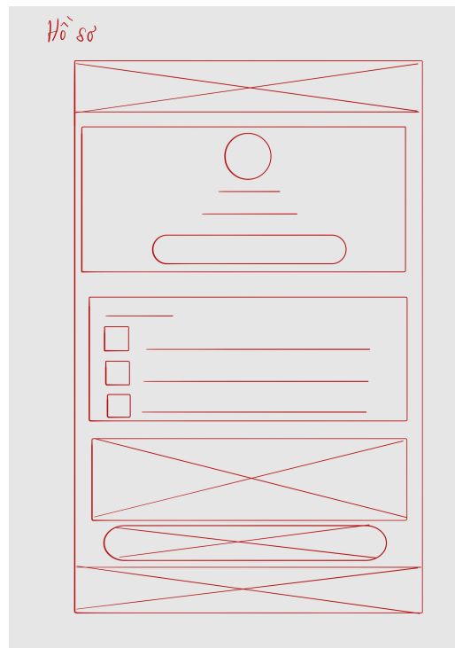
Hình 19: Thiết kế giao diện cho UC9: Quản lý hồ sơ cá nhân
