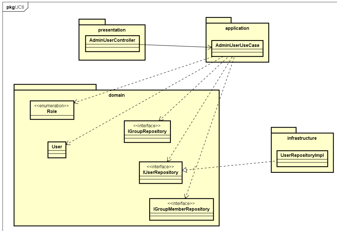
Hình 50: Biểu đồ gói chi tiết cho UC8: Quản trị người dùng
