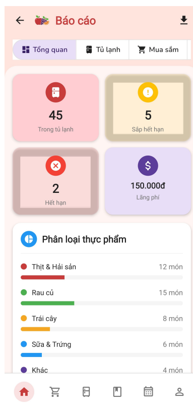
Hình 37: Thiết kế giao diện thống kê và báo cáo - 3
