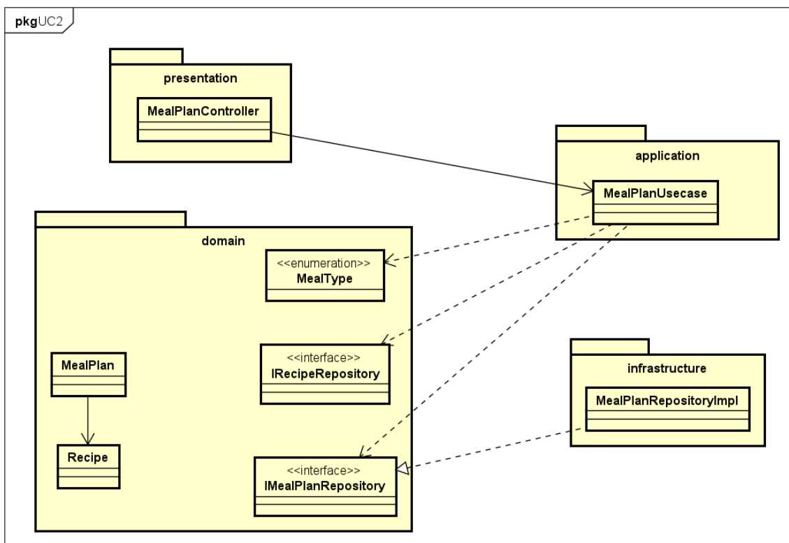
Hình 44: Biểu đồ gói chi tiết cho UC2: Quản lý dự định bữa ăn
