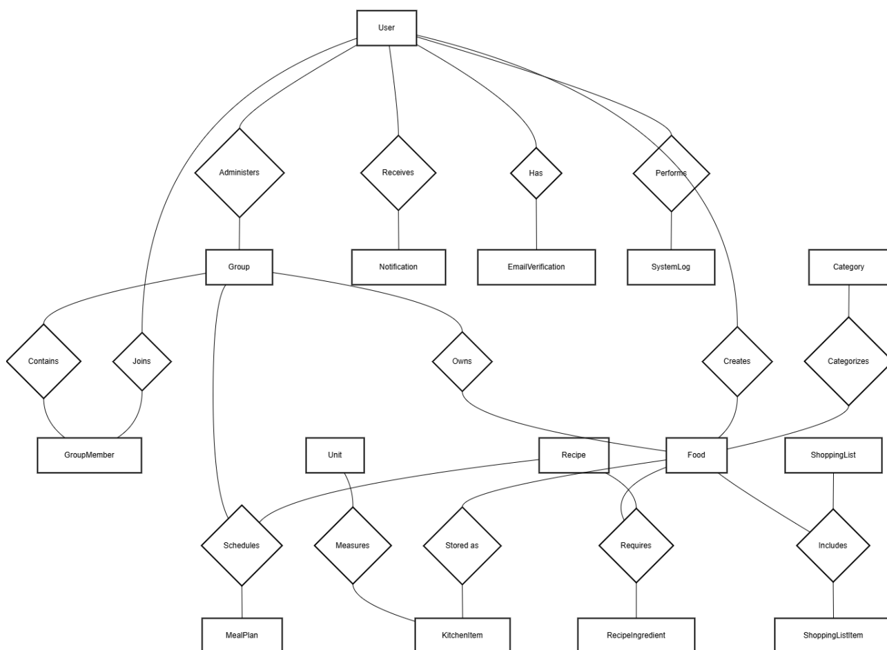
Hình 41: Sơ đồ thực thể quan hệ (ERD) của hệ thống
