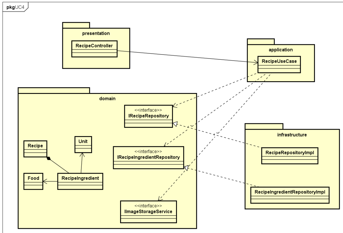
Hình 46: Biểu đồ gói chi tiết cho UC4: Quản lý công thức nấu ăn
