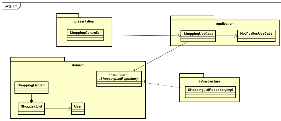
Hình 43: Biểu đồ gói chi tiết cho UC1: Quản lý danh sách mua sắm
