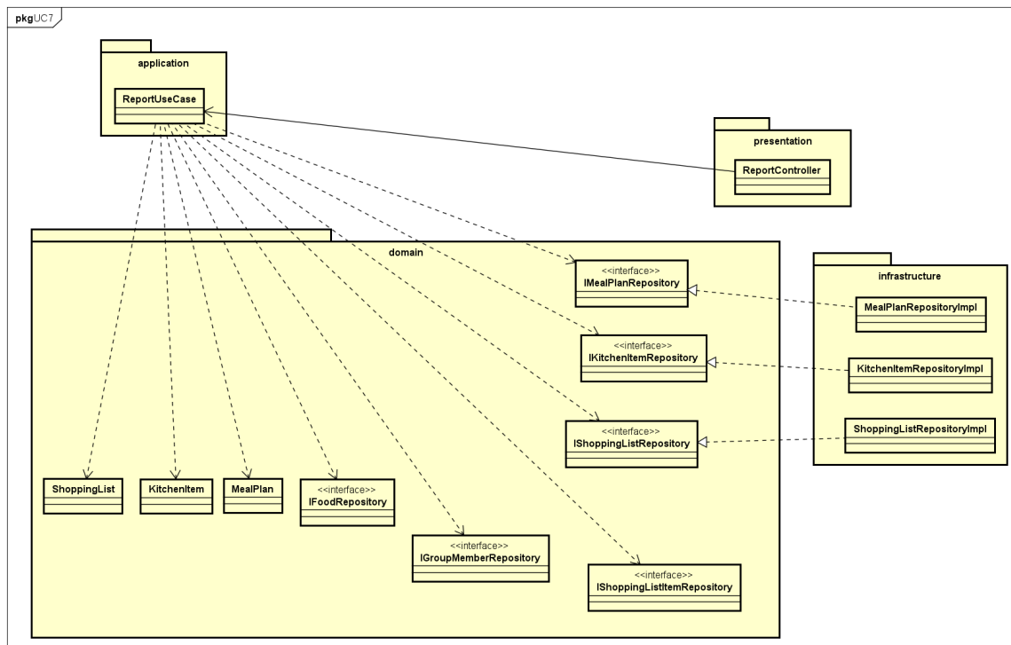
Hình 49: Biểu đồ gói chi tiết cho UC7: Thống kê và báo cáo
