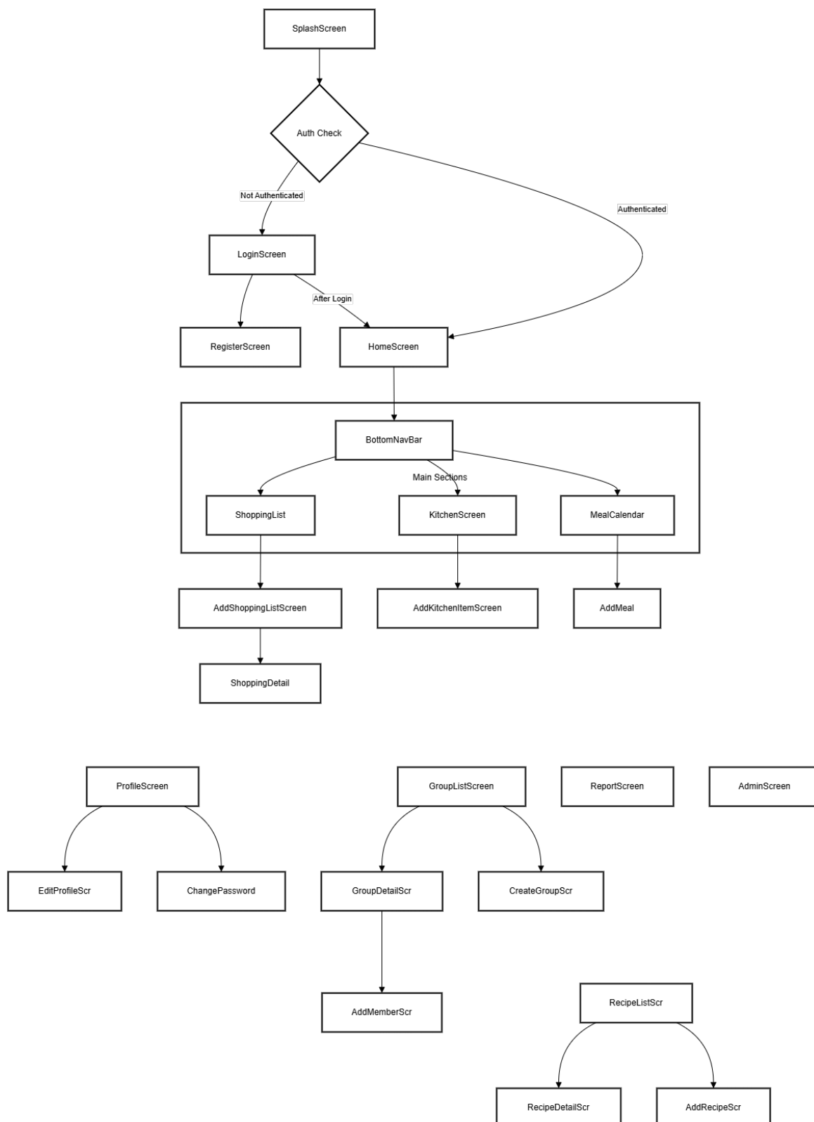
Hình 20: Sơ đồ điều hướng của ứng dụng
