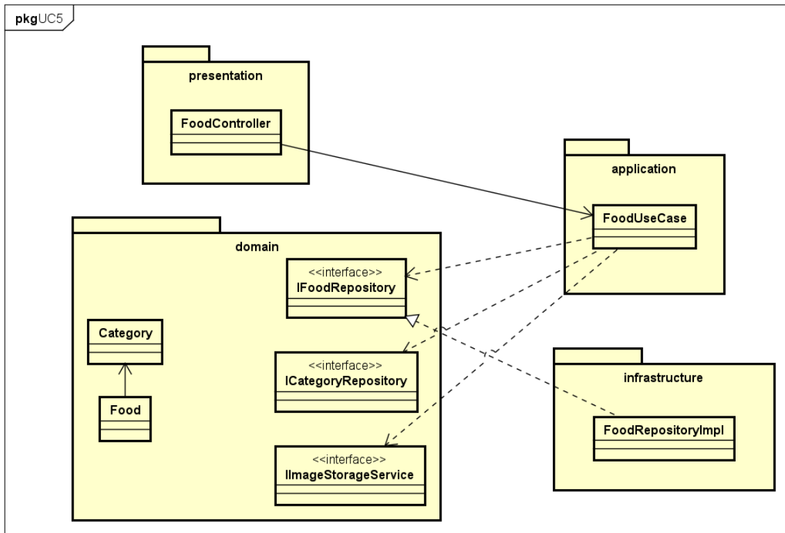
Hình 47: Biểu đồ gói chi tiết cho UC5: Quản lý danh sách thực phẩm
