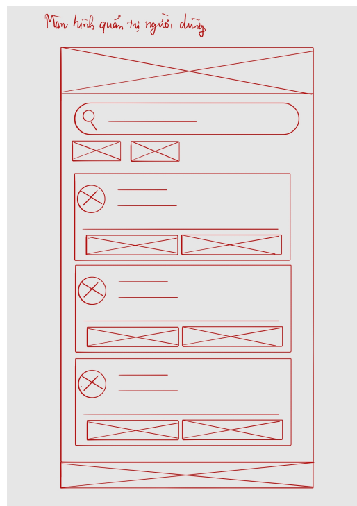
Hình 17: Thiết kế giao diện cho UC8: Quản trị người dùng
