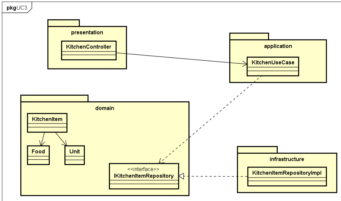
Hình 45: Biểu đồ gói chi tiết cho UC3: Quản lý thực phẩm trong bếp
