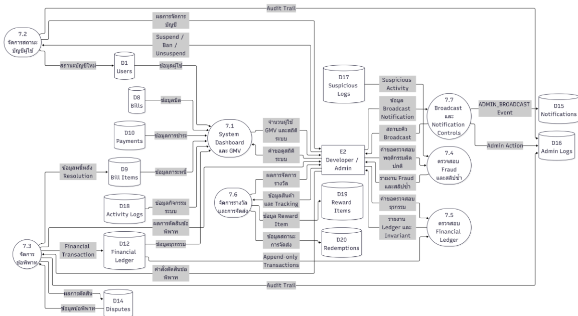
ภาพที่ 3.13 แผนภาพ DFD Level 2 Process 7 ระบบแพคเกจควบคุมสำหรับผู้ดูแลระบบและนักพัฒนา
