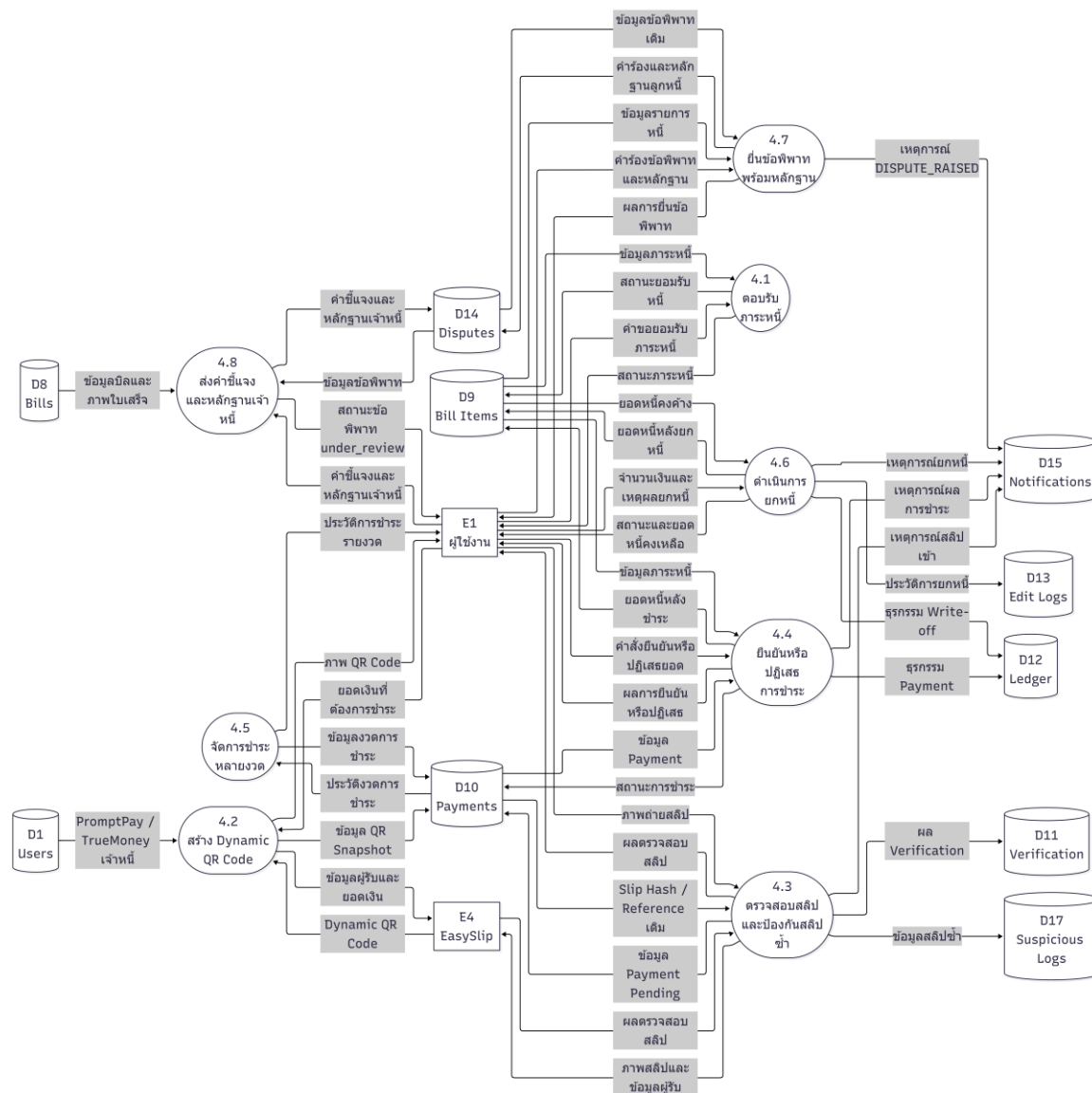
ภาพที่ 3.10 แผนภาพ DFD Level 2 Process 4 ระบบการชำระเงินผ่านพร้อมเพย์และตรวจสอบสลิป
