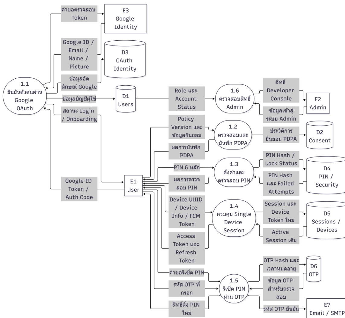
ภาพที่ 3.7 แผนภาพ DFD Level 2 Process 1 กระบวนการพิสูจน์ตัวตนเพื่อยืนยันว่าผู้ใช้งานเป็นบุคคลที่ได้รับอนุญาตจริงก่อนเข้าสู่ระบบหรือแอปพลิเคชัน
