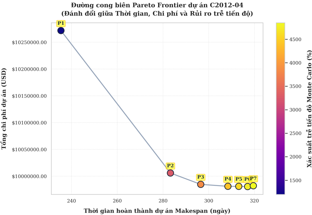
Hình 3.9. Biểu đồ đường cong Pareto Frontier thể hiện sự đánh đổi giữa Thời gian, Chi phí và Rủi ro trễ hạn
