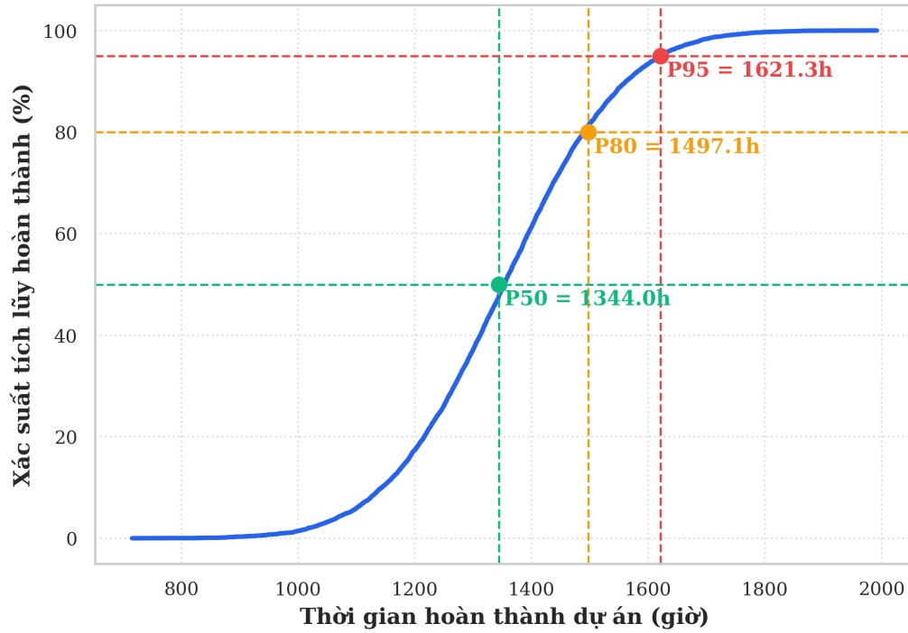
Hình 3.5. Đường cong phân phối xác suất tích lũy CDF thời lượng dự án từ mô phỏng Monte Carlo CPM
