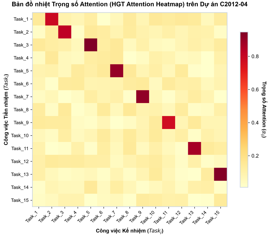
Hình 3.4. Bản đồ nhiệt trọng số Attention định vị các nút công việc tới hạn trên Dự án C2012-04
