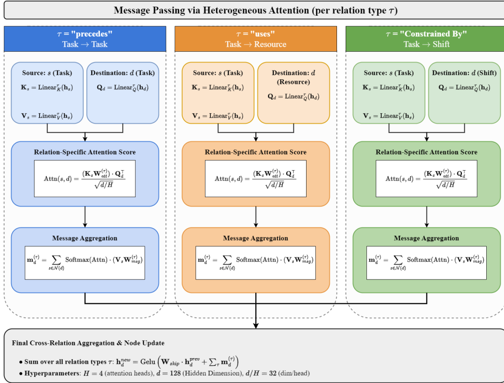
Hình 1.9. Cơ chế tính toán Attention chi tiết trên các quan hệ dị thể trong lớp HGTConv.
