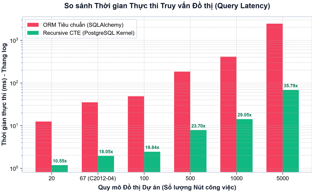
Hình 3.10. Biểu đồ cột so sánh thời gian thực thi truy vấn đồ thị giữa ORM tiêu chuẩn và Recursive CTE
