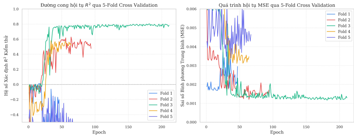
Hình 3.3. Đường cong học tập đánh giá quá trình hội tụ Loss và R^2 Score qua 5-Fold Cross Validation
