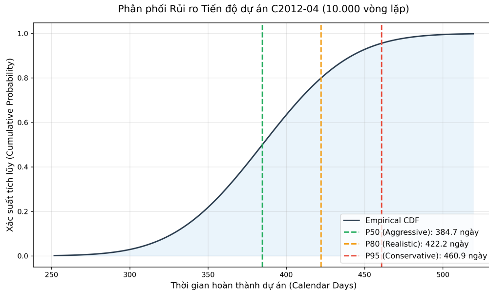
Hình 3.5. Đường cong phân phối tích lũy CDF mô phỏng Monte Carlo CPM (10.000 vòng lặp, Dự án C2012-04)
