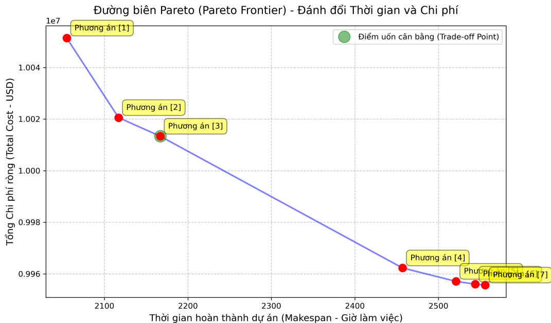
Hình 3.7. Đường biên Pareto thể hiện sự đánh đổi Thời gian - Chi phí
