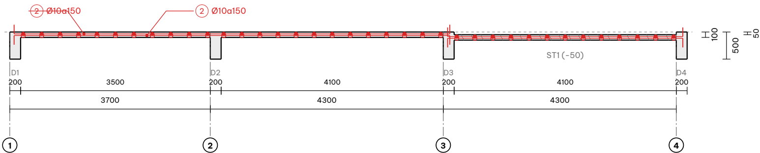
MẶT CẮT THÉP SÀN B-B
