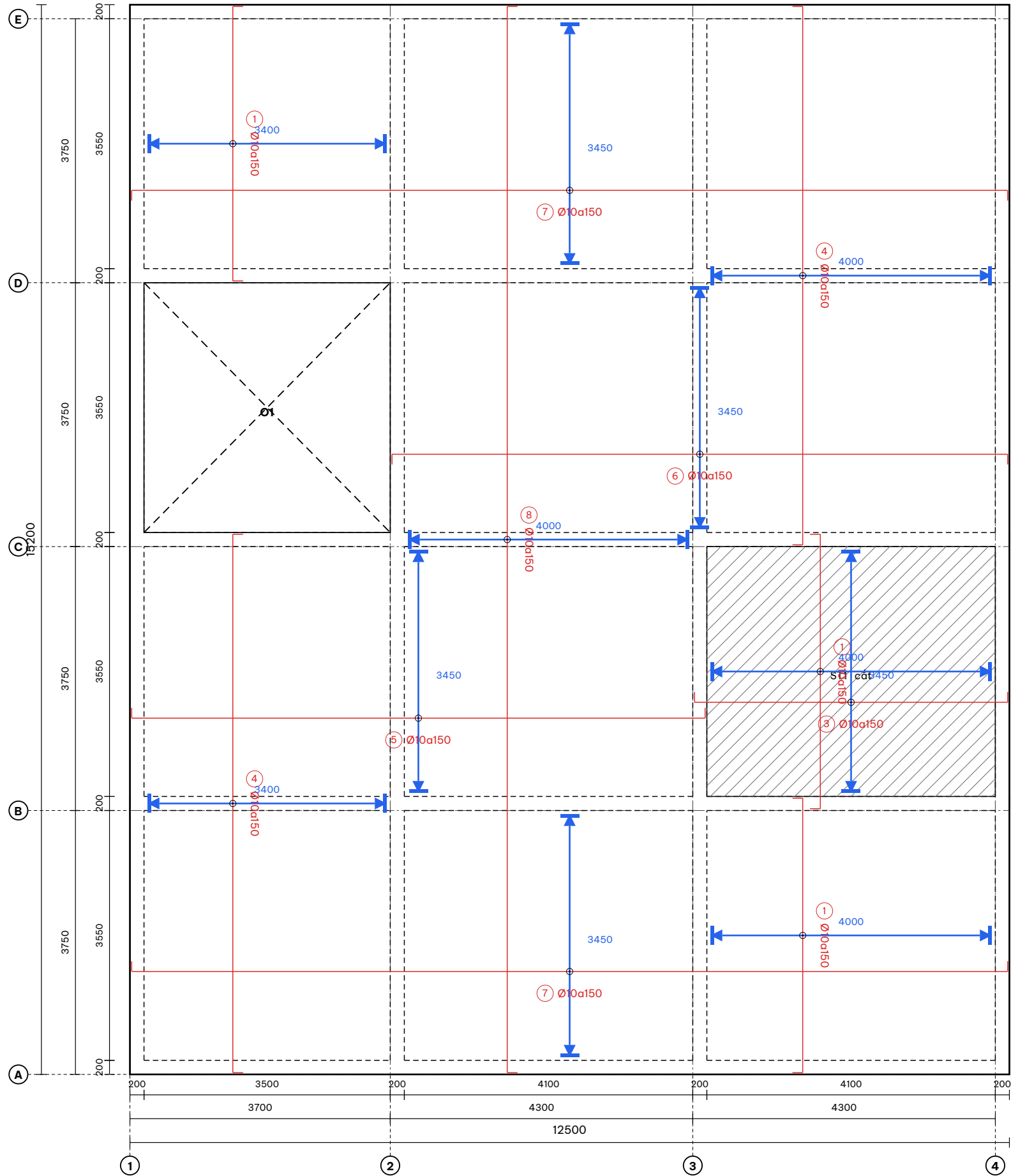
MẶT BẰNG CỐT THÉP SÀN LỚP DƯỚI TL: 1/100
