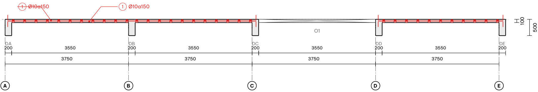
MẶT CẮT THÉP SÀN A-A
