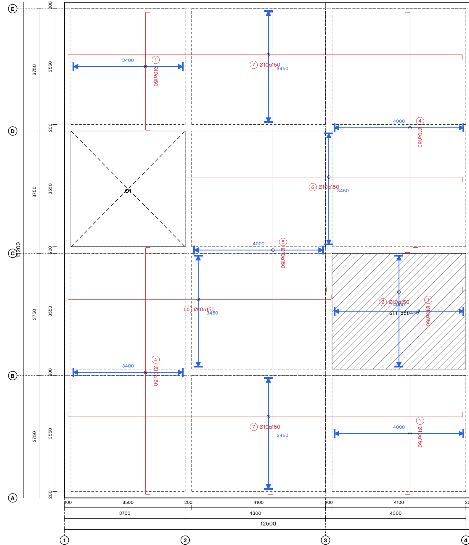
MẶT BẰNG CỐT THÉP SÀN LỚP TRÊN TL: 1/100
