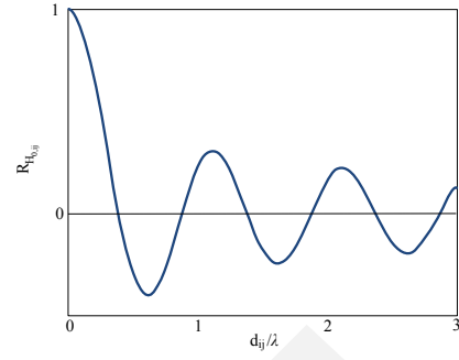
Figura 18. Coefficiente di correlazione spaziale al variare della distanza tra antenne equipolarizzate.
