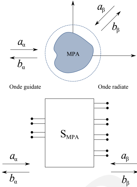
Figura 12. MPA e rappresentazione modale della propagazione elettromagnetica tra guidata e radiata.
