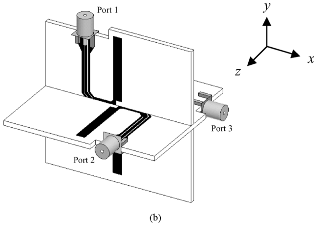
Figura 20. MPoA di tre dipoli stampati progettato per sistemi MIMO.
