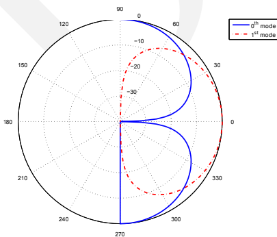
Figura 22. Pattern relativo all'MMA di Fig. 21.
