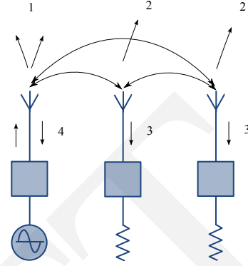
Figura 17. Meccanismi fisici in un MPA: 1. Radiazione, 2. Scattering da elementi non eccitati, 3. Potenza accoppiata, 4. Potenza riflessa
