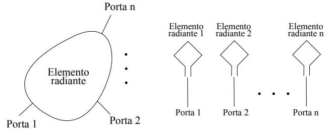
Figura 3. Schematizzazione di Multimode antenna (sinistra) e Multielement antenna (destra).
