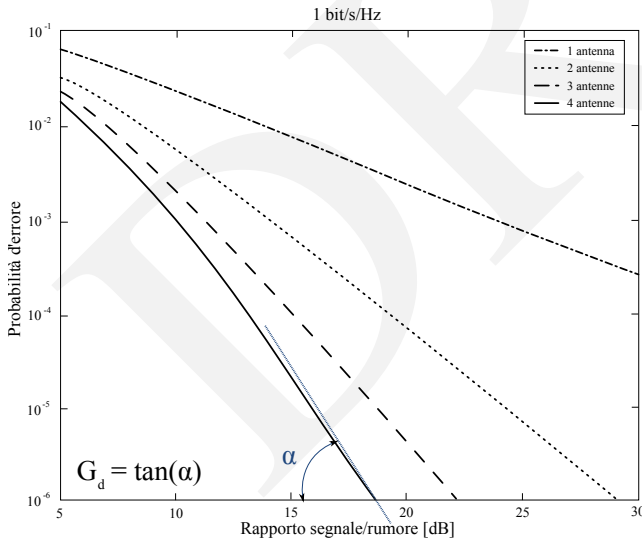
Figura 9. Andamento della probabilità di errore rispetto all'SNR per un sistema STC al variare del numero di antenne in ricezione.
