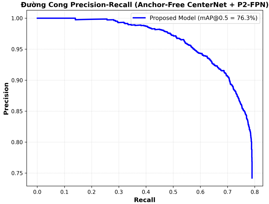
Hình 11: Đường cong Precision-Recall của mô hình đề xuất trên tập kiểm thử Anti-UAV (mAP@0.5 = 76.31%, Precision = 99.85% tại ngưỡng Conf \geq 0.4 ).
