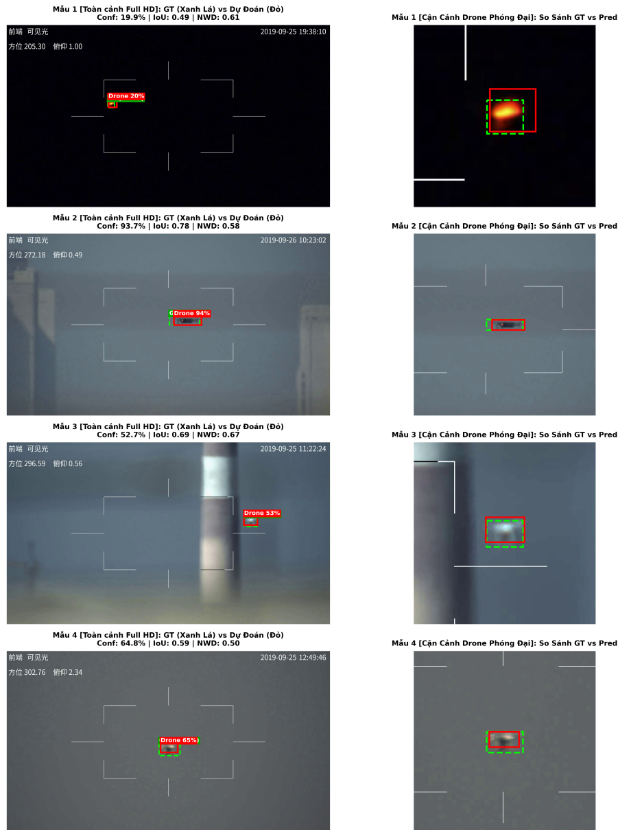
Hình 13: So sánh trực quan chi tiết giữa hộp boc dự đoán (Prediction – viền đỏ liền) và nhân thực tế (Ground Truth – viền xanh lá nét đứt) trên các mẫu kiểm thử Anti-UAV trong điều kiện toàn cảnh và phóng đại cận cảnh.
