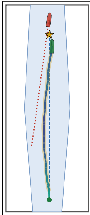
(d) overtaking — channel min. range 3.19 m, goal
