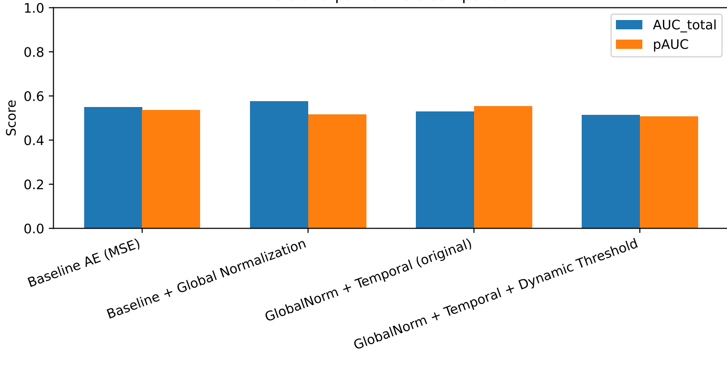
AUC and partial AUC comparison
