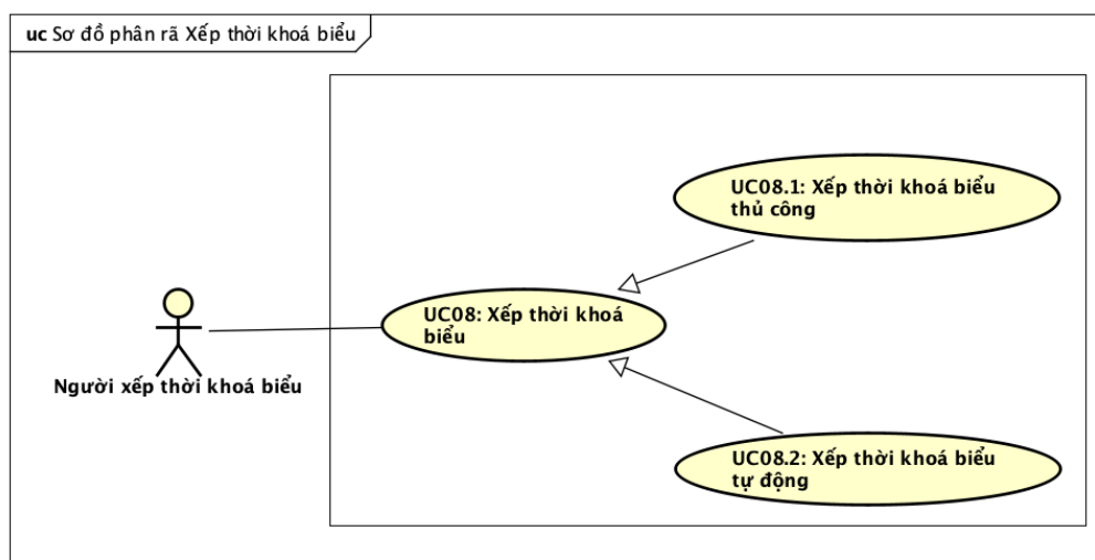
Hình 2.3: Biểu đồ ca sử dụng phân rã xếp thời khoá biểu
