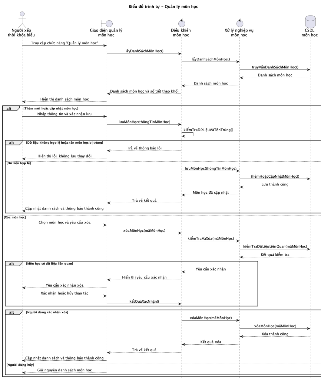
Hình 2.5: Biểu đồ tuần tự ca sử dụng Quản lý môn học
