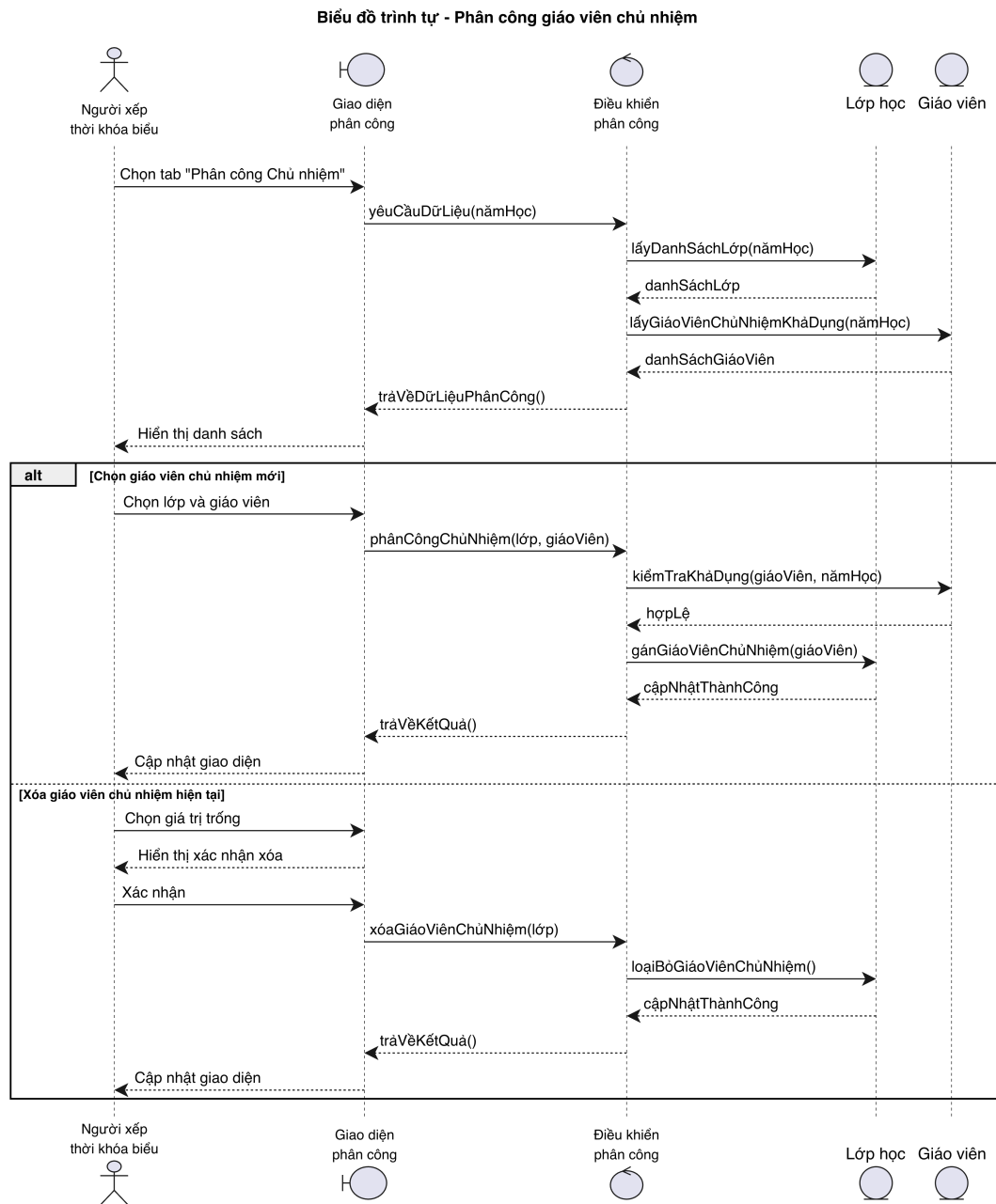
Hình 2.10: Biểu đồ tuần tự ca sử dụng Phân công giáo viên chủ nhiệm
