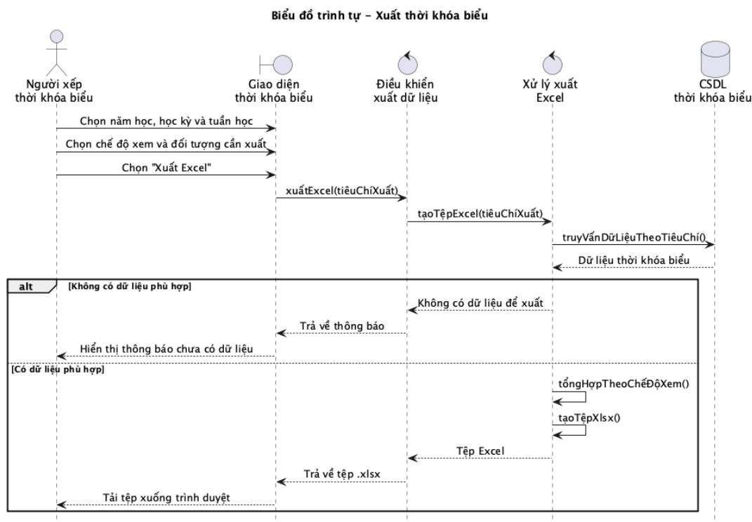
Hình 2.15: Biểu đồ tuần tự ca sử dụng Xuất thời khoá biểu
