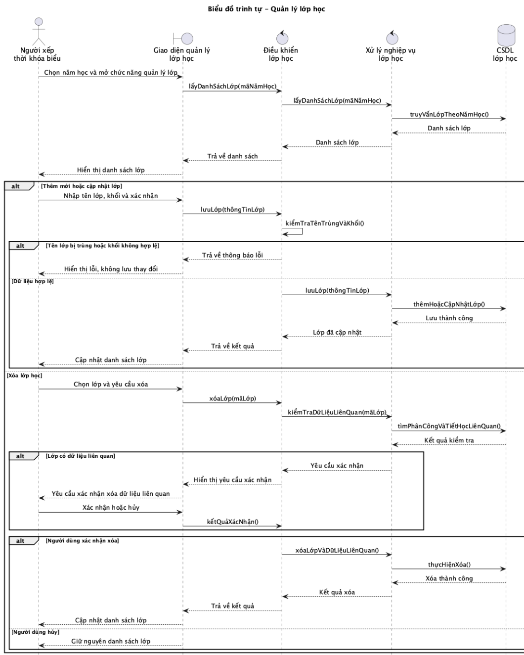
Hình 2.9: Biểu đồ tuần tự ca sử dụng Quản lý lớp học
