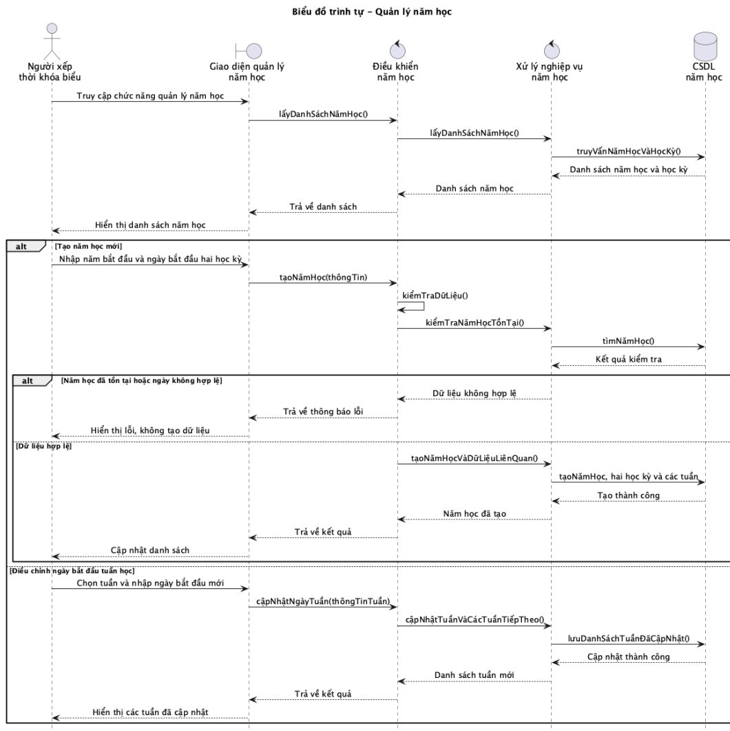
Hình 2.8: Biểu đồ tuần tự ca sử dụng Quản lý năm học
