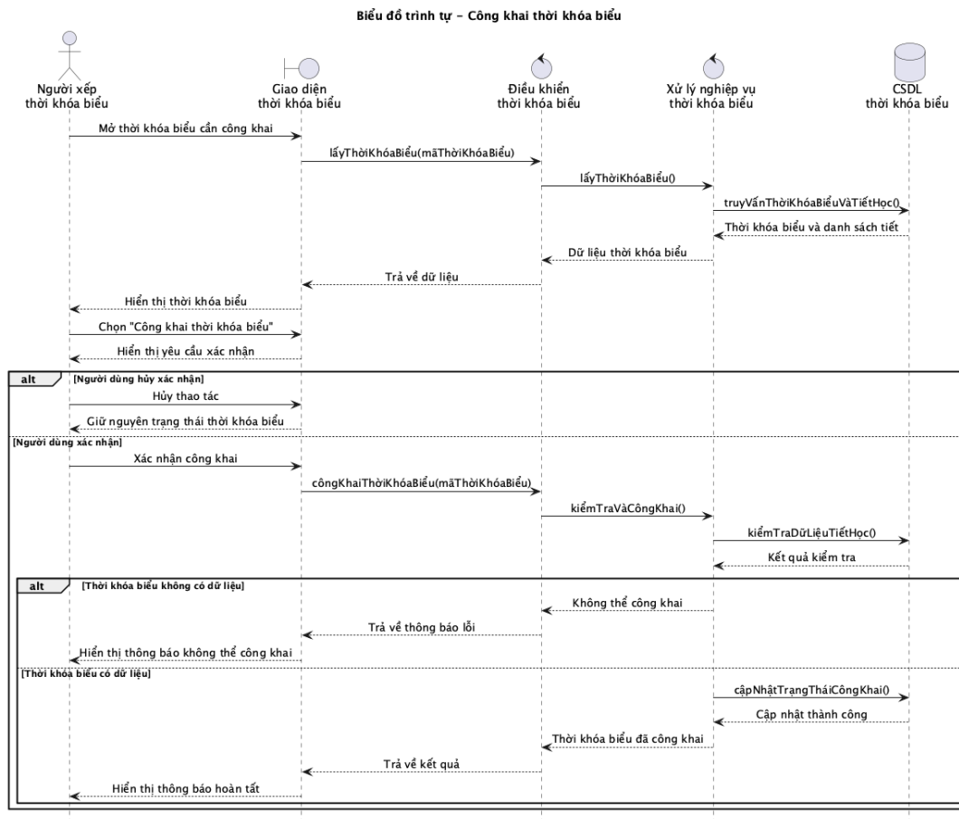
Hình 2.14: Biểu đồ tuần tự ca sử dụng Công khai thời khoá biểu
