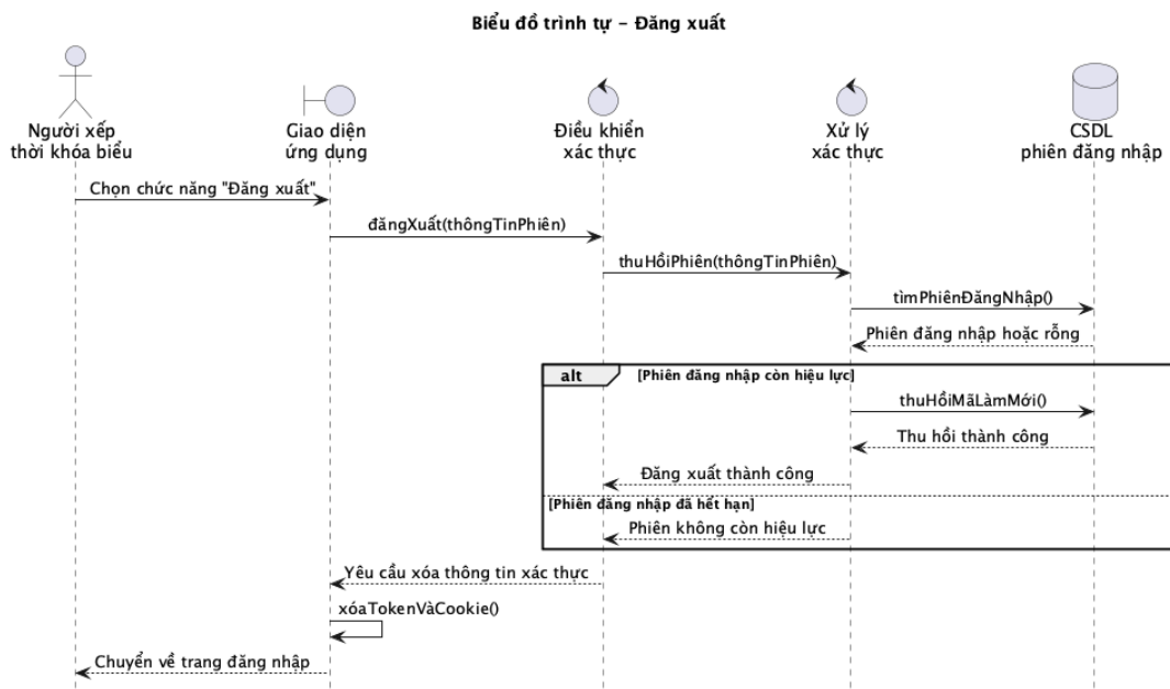
Hình 2.16: Biểu đồ tuần tự ca sử dụng Đăng xuất
