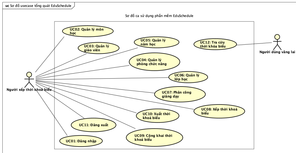
Hình 2.1: Biểu đồ ca sử dụng hệ thống
