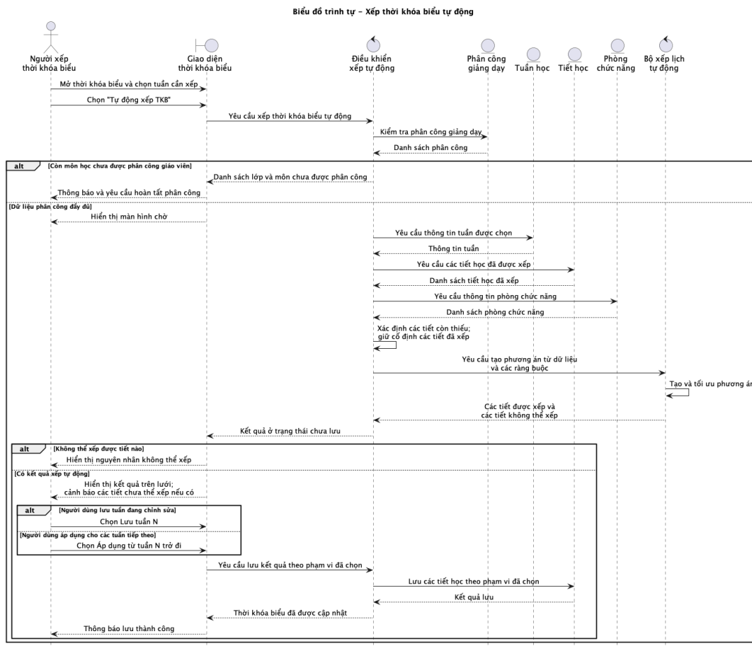
Hình 2.13: Biểu đồ tuần tự ca sử dụng Xếp thời khoá biểu tự động
