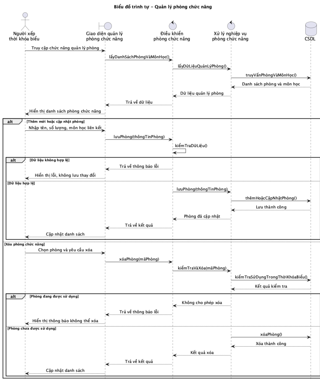
Hình 2.7: Biểu đồ tuần tự ca sử dụng Quản lý phòng chức năng
