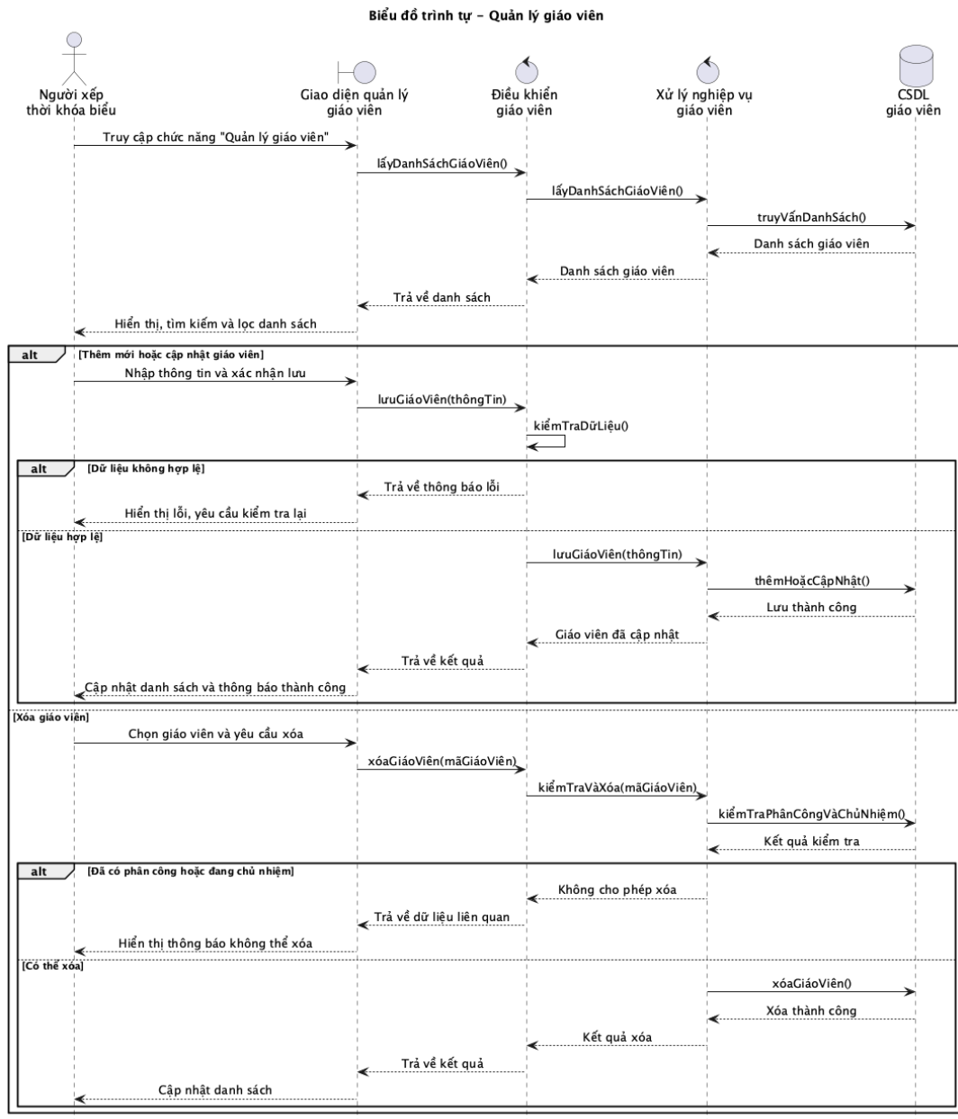
Hình 2.6: Biểu đồ tuần tự ca sử dụng Quản lý giáo viên
