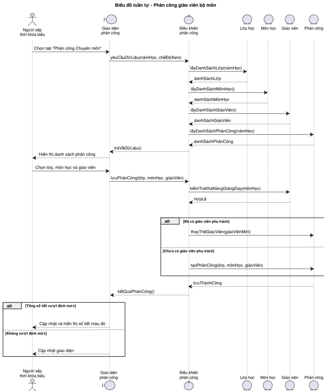
Hình 2.11: Biểu đồ tuần tự ca sử dụng Phân công giáo viên bộ môn
