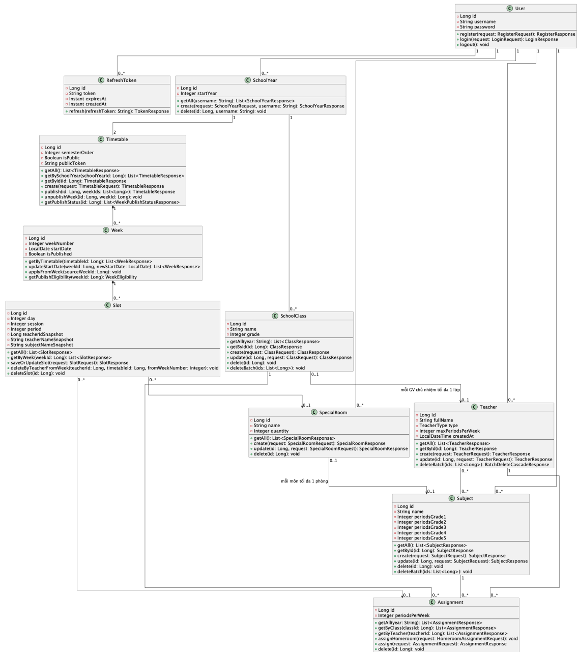
Hình 4.3: Biểu đồ lớp thiết kế của hệ thống EduSchedule
