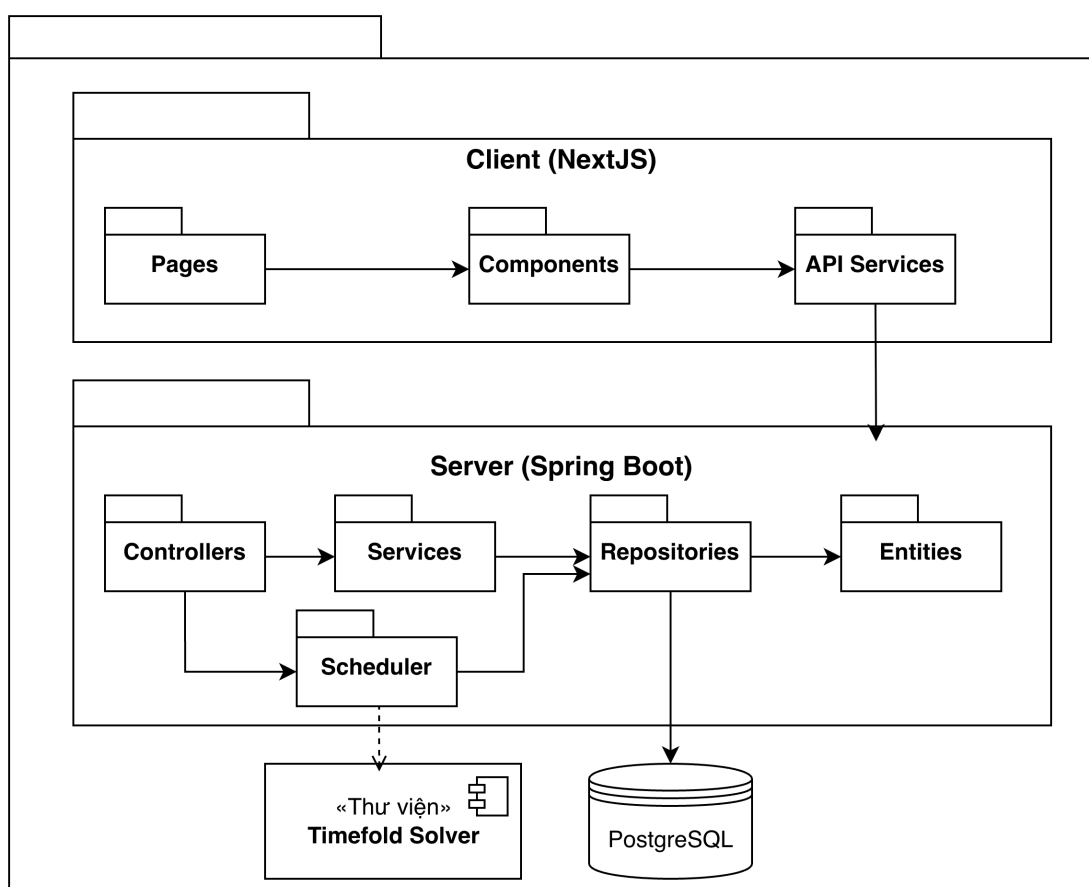
Hình 4.2: Biểu đồ gói tổng quan của hệ thống EduSchedule
