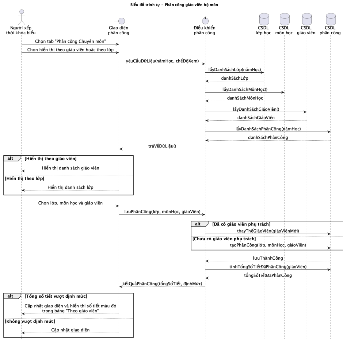
Hình 2.11: Biểu đồ tuần tự ca sử dụng Phân công giáo viên bộ môn
