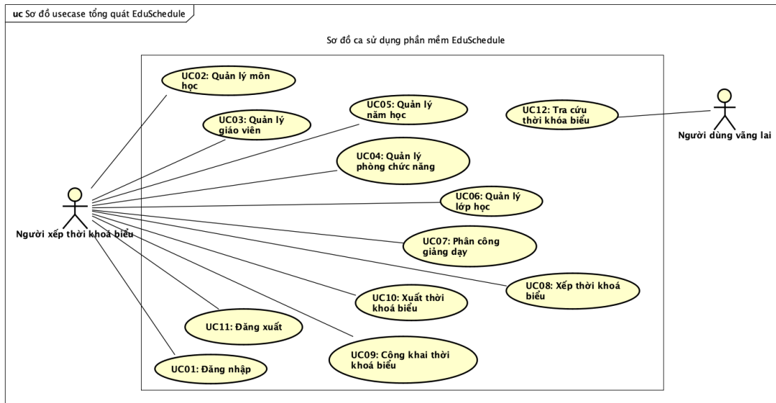
Hình 2.1: Biểu đồ ca sử dụng hệ thống
