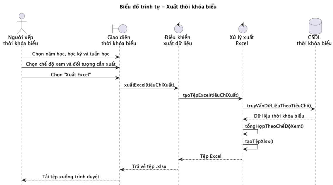
Hình 2.15: Biểu đồ tuần tự ca sử dụng Xuất thời khoá biểu
