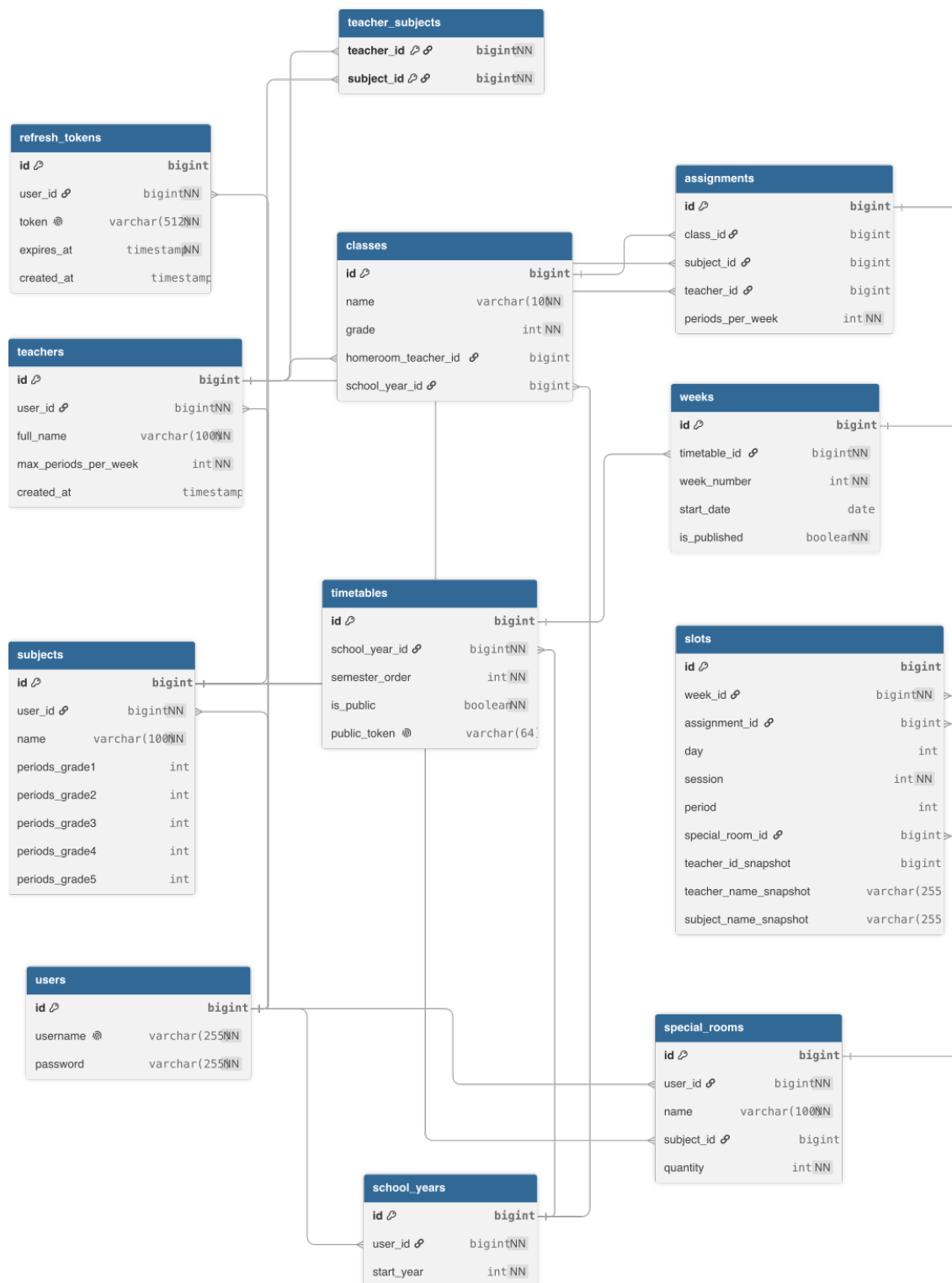
Hình 4.4: Thiết kế cơ sở dữ liệu cho hệ thống EduSchedule
