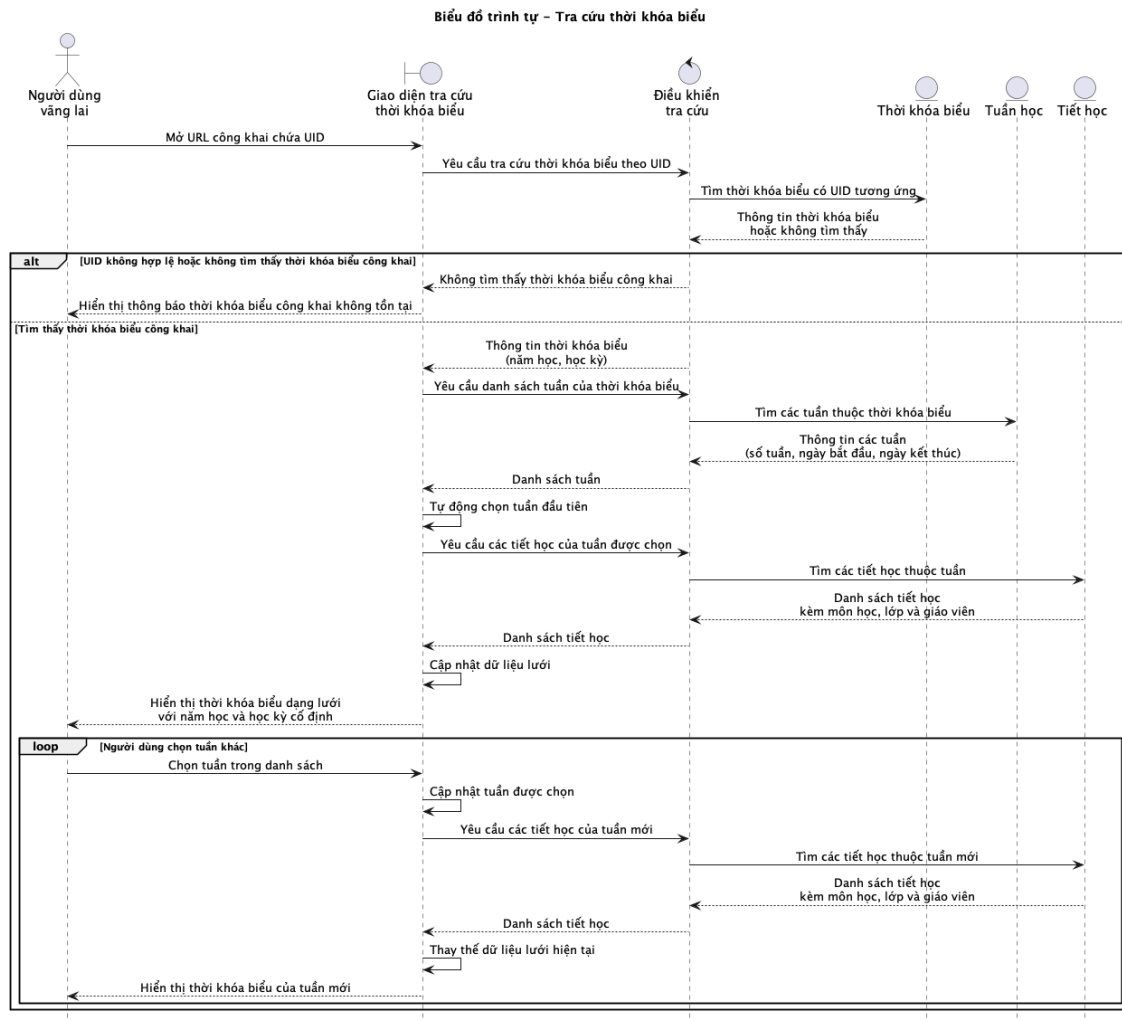
Hình 2.17: Biểu đồ tuần tự ca sử dụng Tra cứu thời khoá biểu
