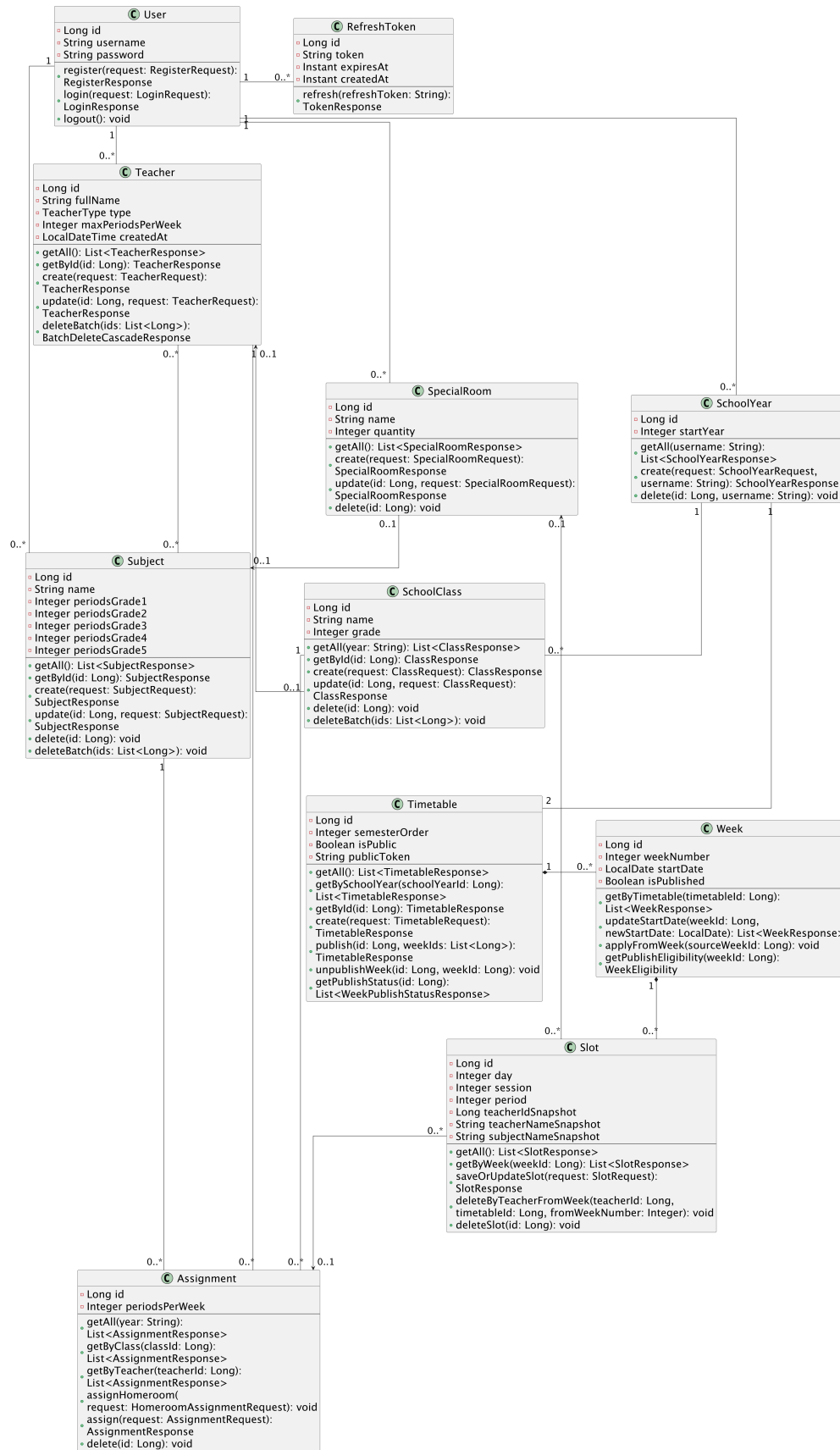
Hình 4.3: Biểu đồ lớp thiết kế của hệ thống EduSchedule
