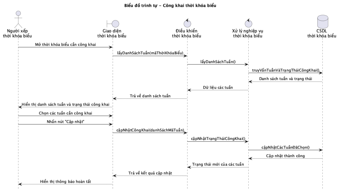
Hình 2.14: Biểu đồ tuần tự ca sử dụng Công khai thời khoá biểu
