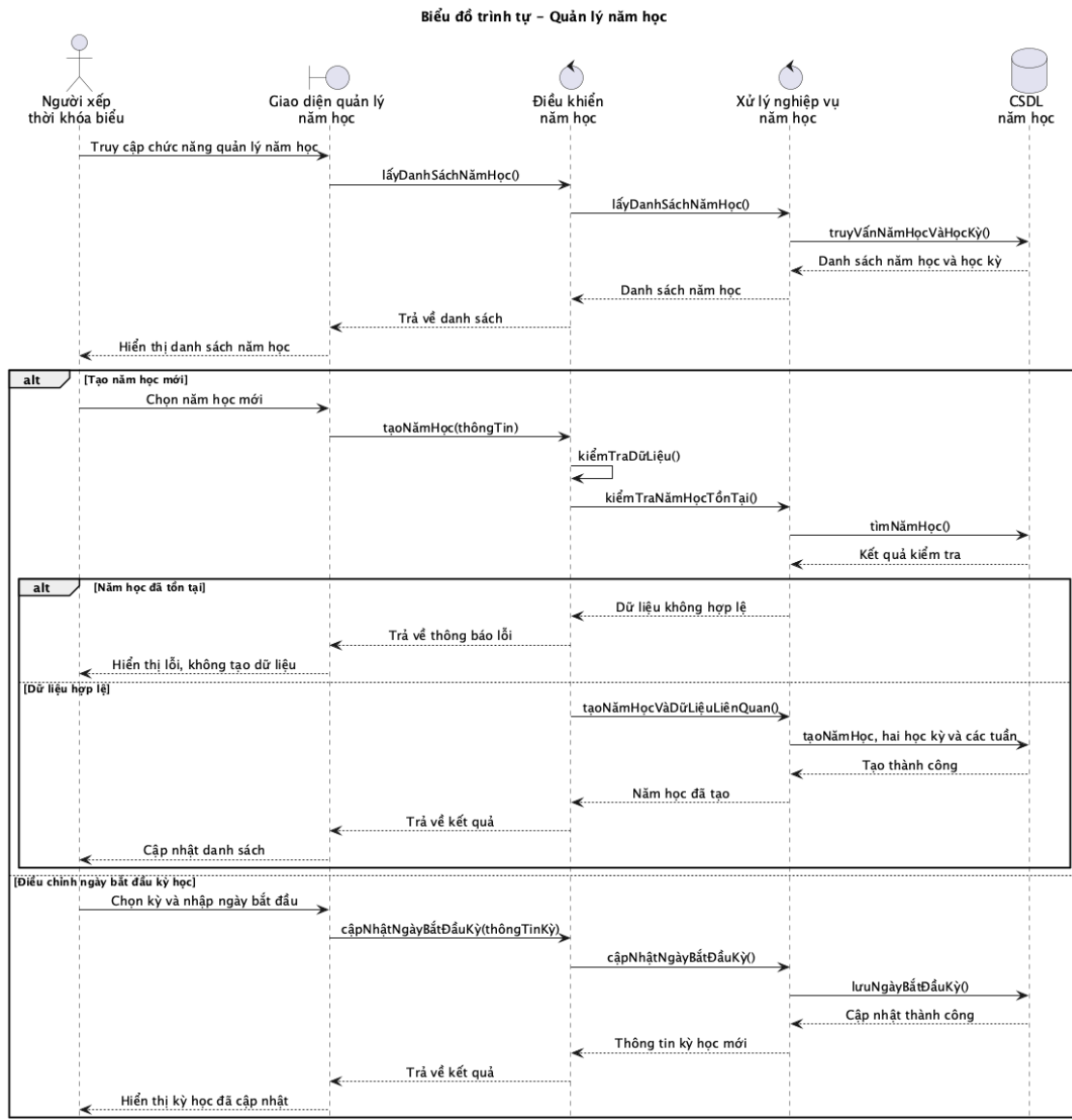
Hình 2.8: Biểu đồ tuần tự ca sử dụng Quản lý năm học
