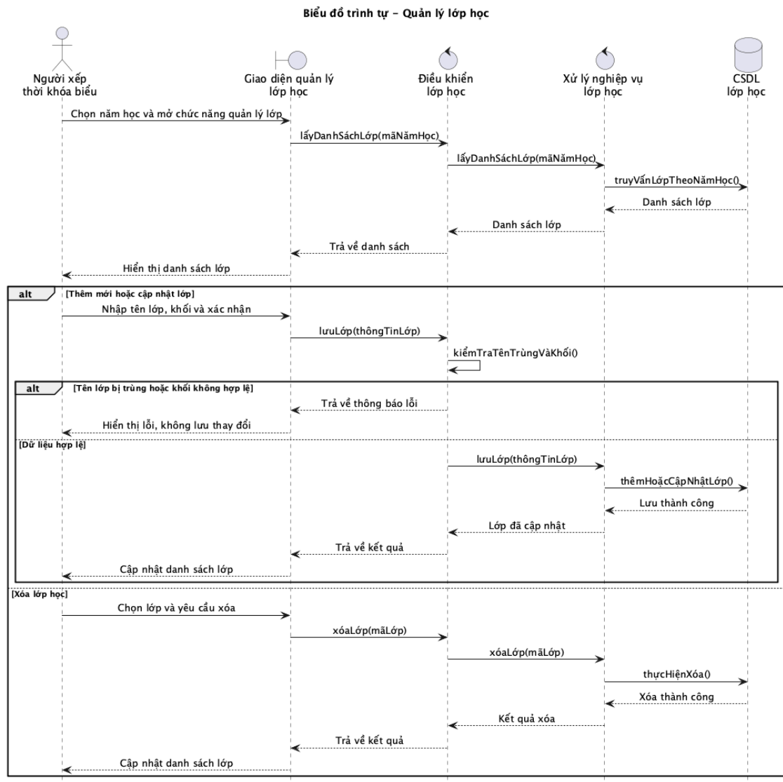
Hình 2.9: Biểu đồ tuần tự ca sử dụng Quản lý lớp học
