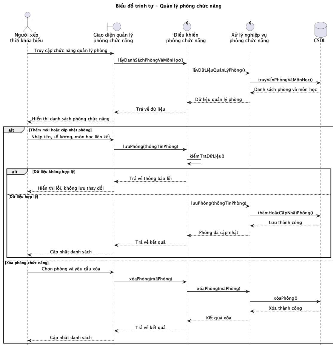
Hình 2.7: Biểu đồ tuần tự ca sử dụng Quản lý phòng chức năng
