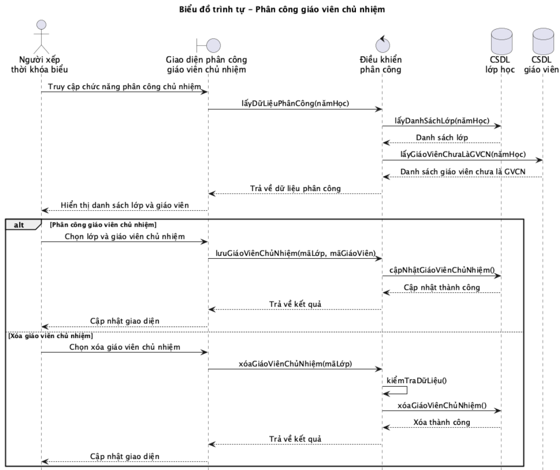
Hình 2.10: Biểu đồ tuần tự ca sử dụng Phân công giáo viên chủ nhiệm
