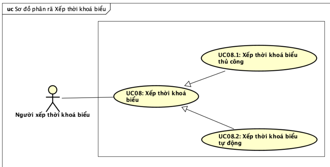
Hình 2.3: Biểu đồ ca sử dụng phân rã xếp thời khóa biểu
