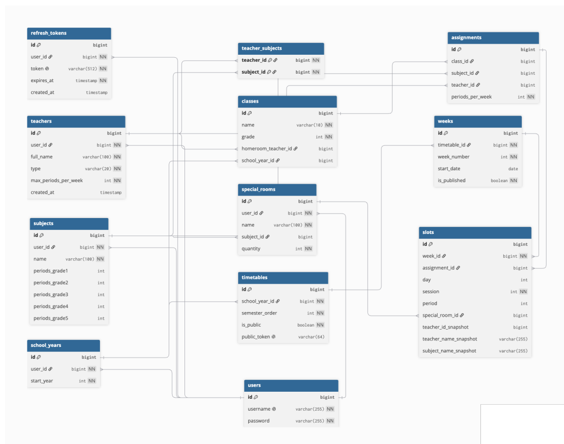
Hình 4.4: Thiết kế cơ sở dữ liệu cho hệ thống EduSchedule
