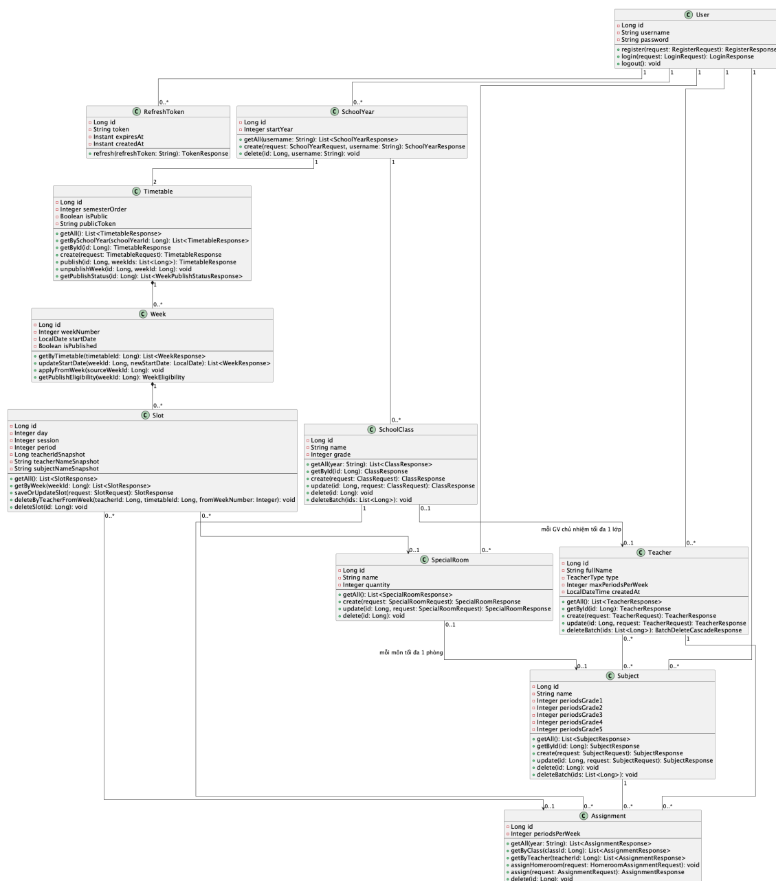
Hình 4.3: Biểu đồ lớp thiết kế của hệ thống EduSchedule
