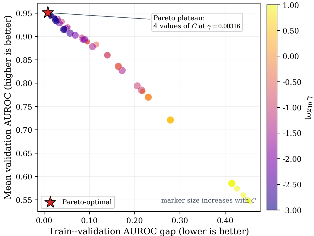
(b) RBF C -- \gamma grid
