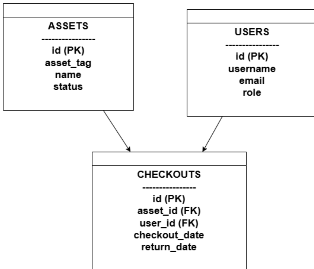
Hình 4.6: Biểu đồ thực thể liên kết của hệ thống
